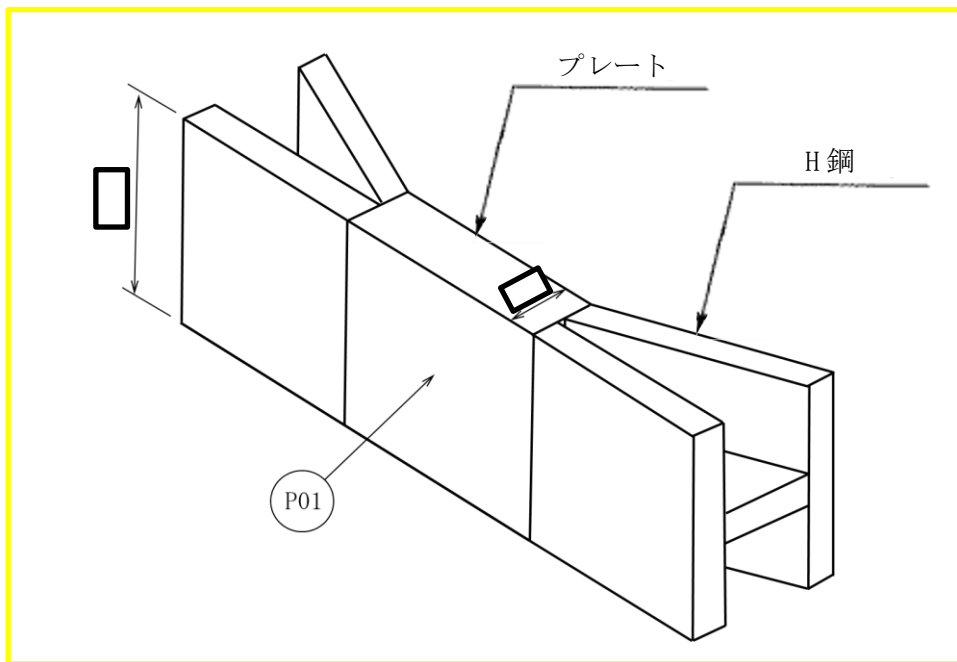
図 3-2 CRD ハウジングレストレントビームの応力評価点 (単位 : mm)
