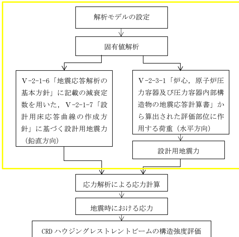
図2-1 CRDハウジングレストレントビームの耐震評価フロー
