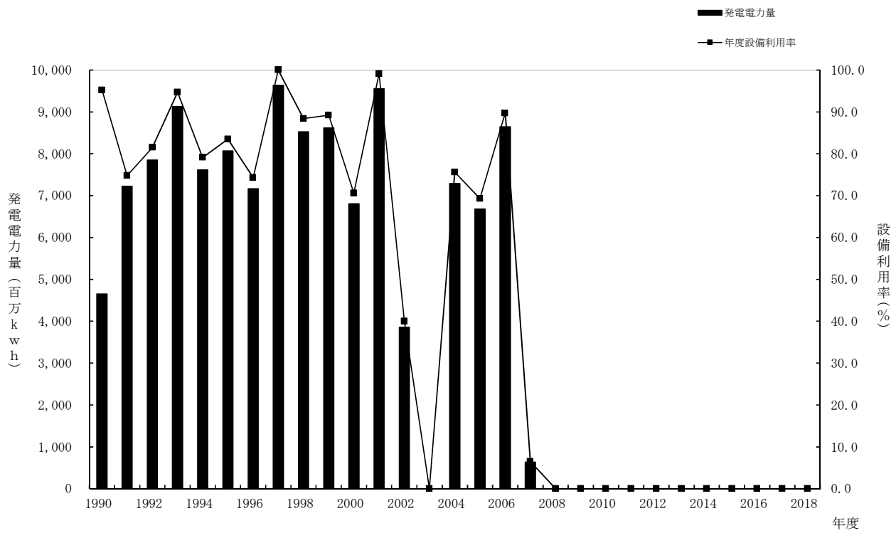
資料 2 - 4 発電電力量・設備利用率の年度推移
