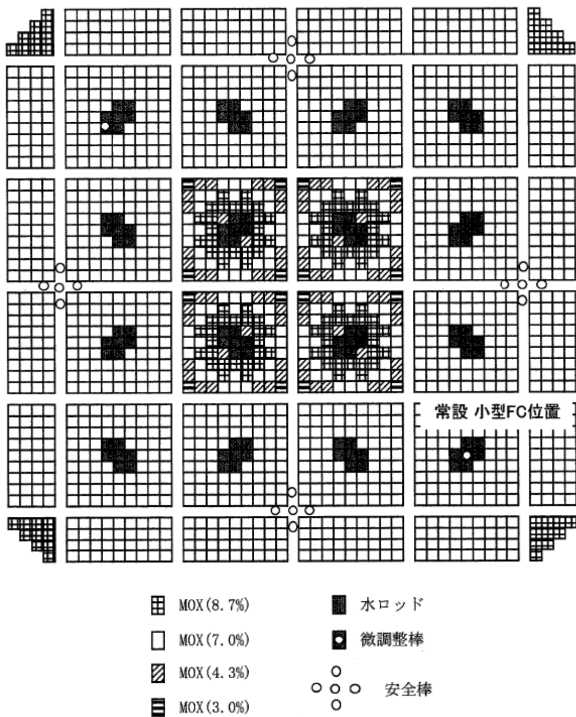
図1 BASALA 試験 (炉心1 : 運転時模擬) ①基準体系試験の炉心図 [2]
