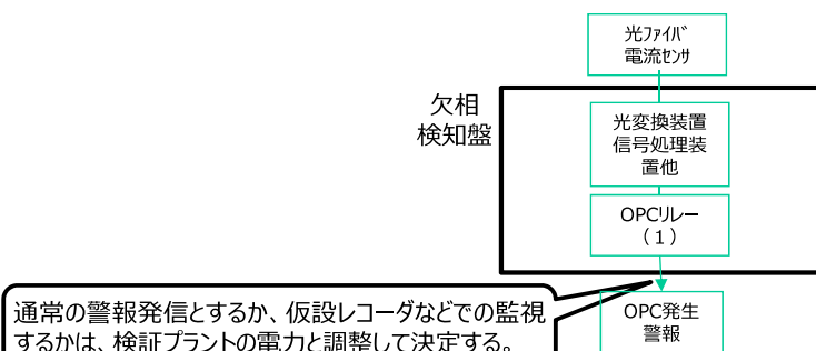
図1 回路構成
