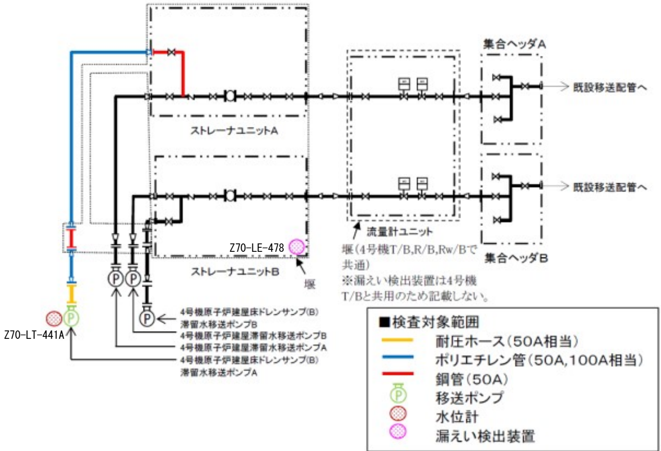
(5) 4号機原子炉建屋床ドレンサンプ(B)から4号機原子炉建屋ストレーナユニット分岐部まで
