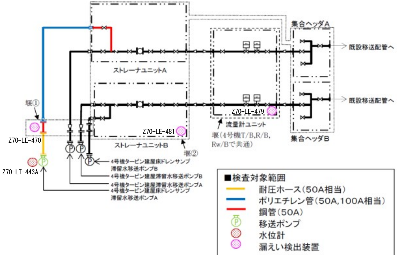
(6) 4号機タービン建屋床ドレンサンプから4号機タービン建屋ストレーナユニット分岐部まで
