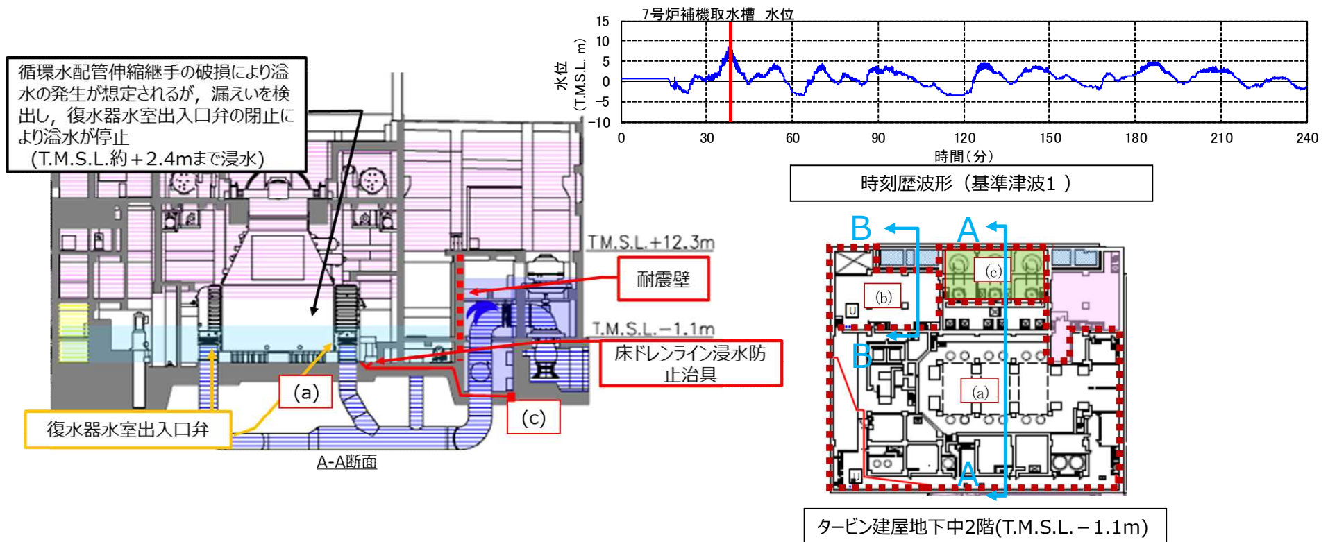
図3：復水器エリアにおける溢水事象
