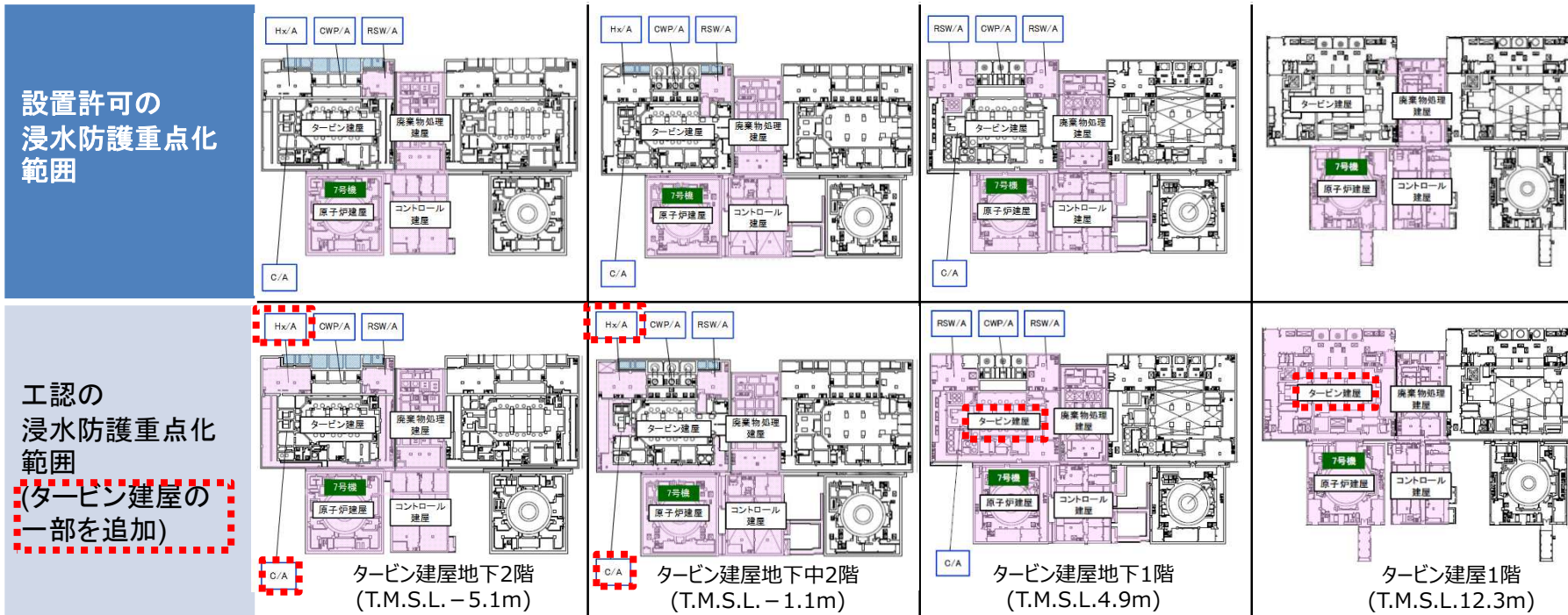
図1：浸水防護重点化範囲
