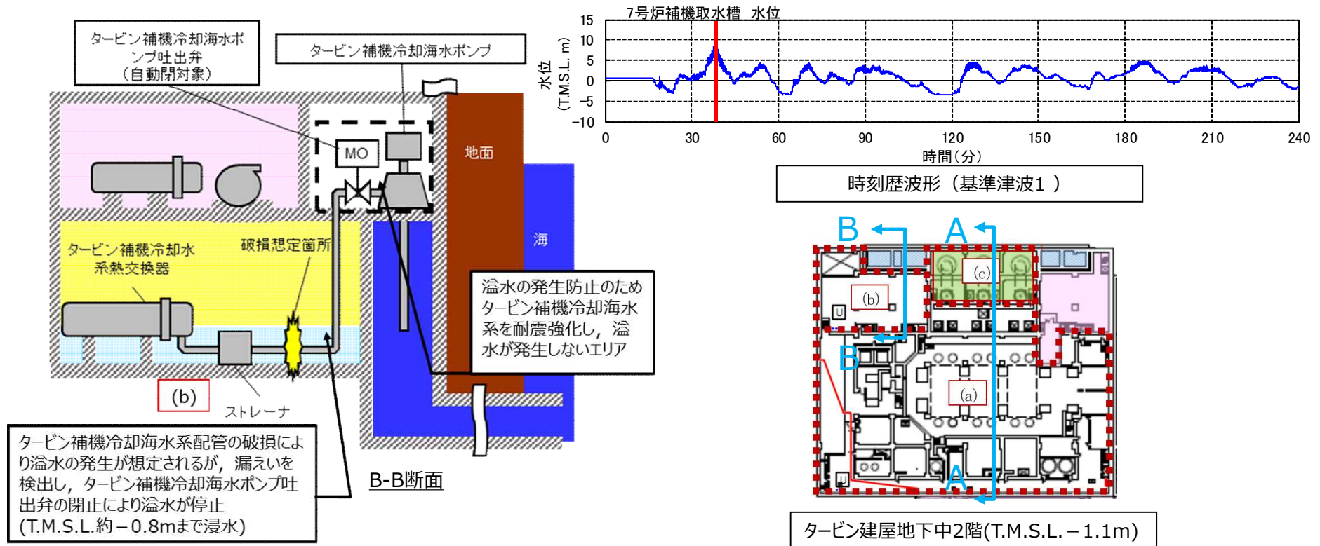
図4：タービン補機冷却系熱交換器エリアにおける溢水事象
