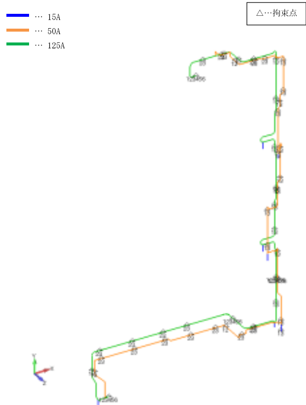
図 4-13-4 配管 (KG84-600) の解析モデル
