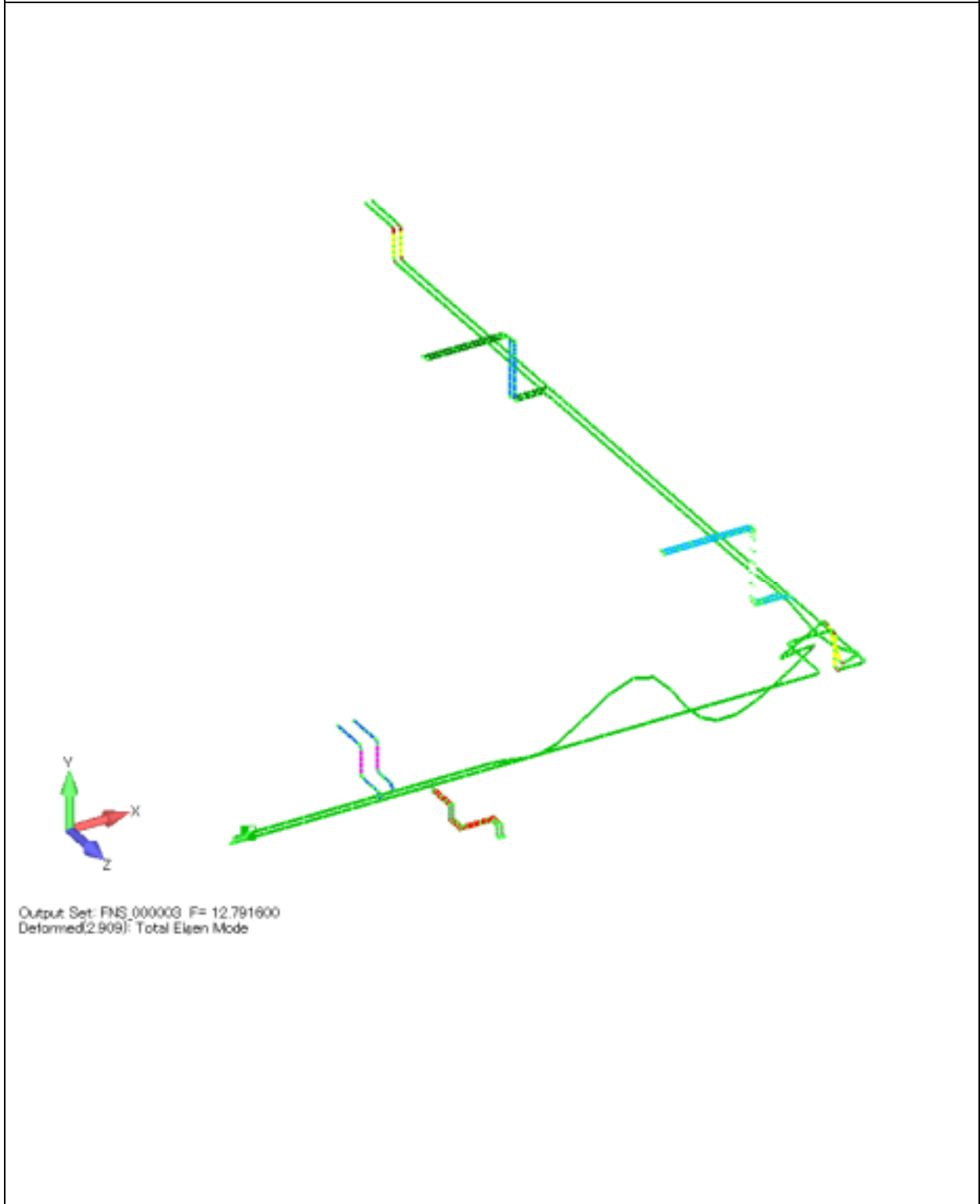
図 4-14-10 配管 (KG84-617) 固有モード図 (3/3)
