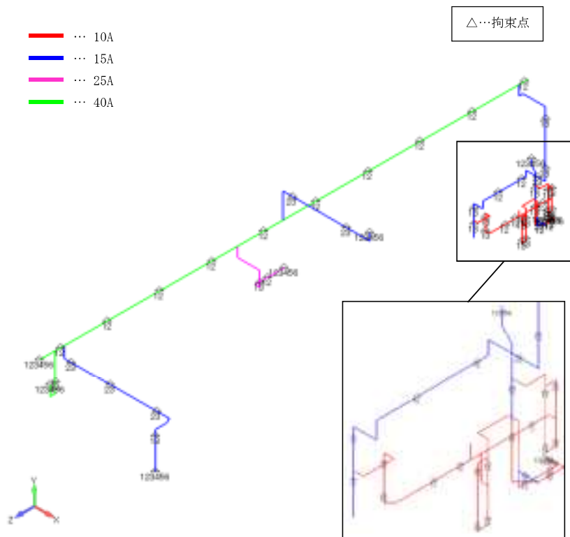
図 4-13-7 配管 (A86IA-1) の解析モデル
