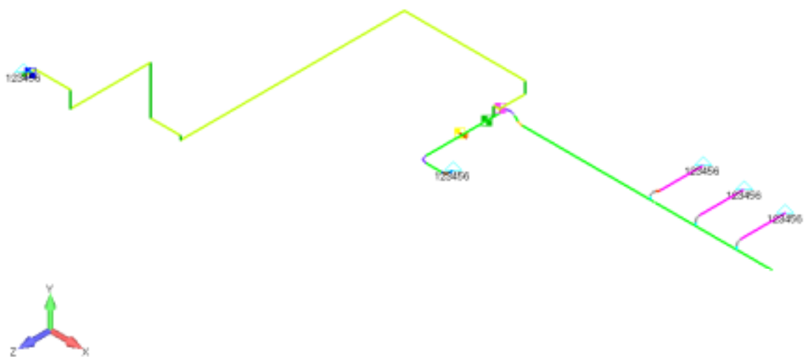
図 4-13-5 配管 (KG83-624) の解析モデル
