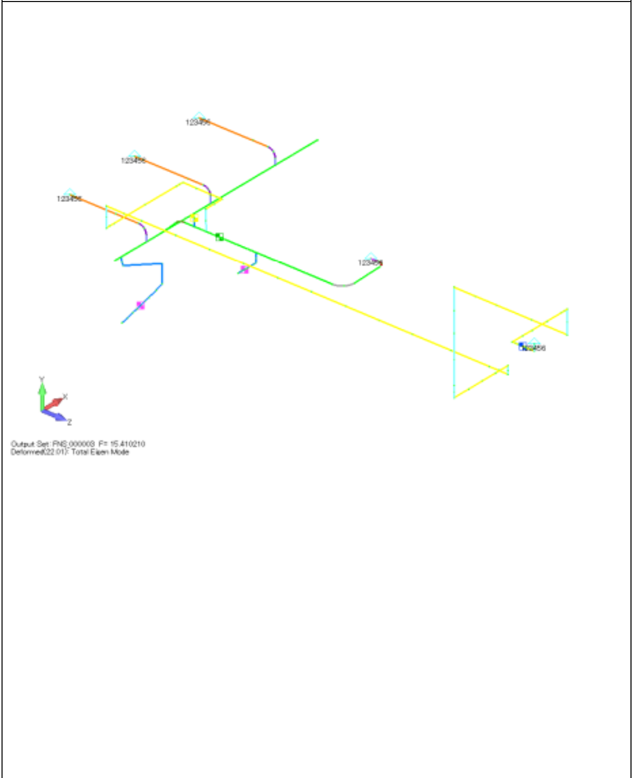
図 4-14-2 配管(KG83-619) 固有モード図 (3/3)
