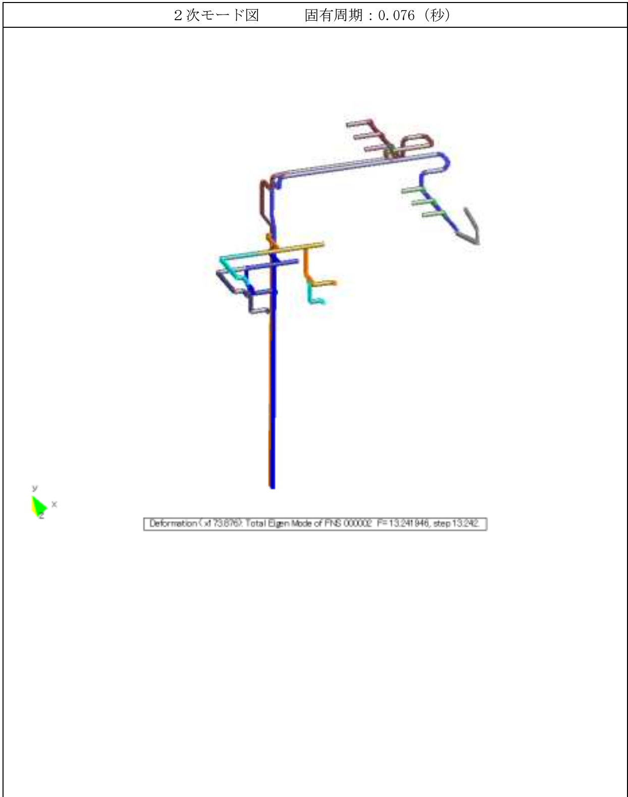
図 4-14-3 配管(KG83-618) 固有モード図 (2/3)
