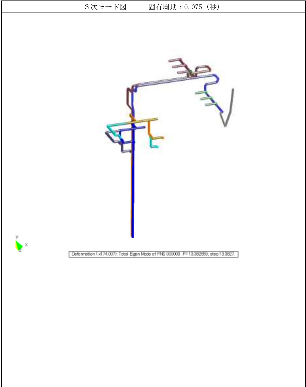
図 4-14-3 配管(KG83-618) 固有モード図 (3/3)
