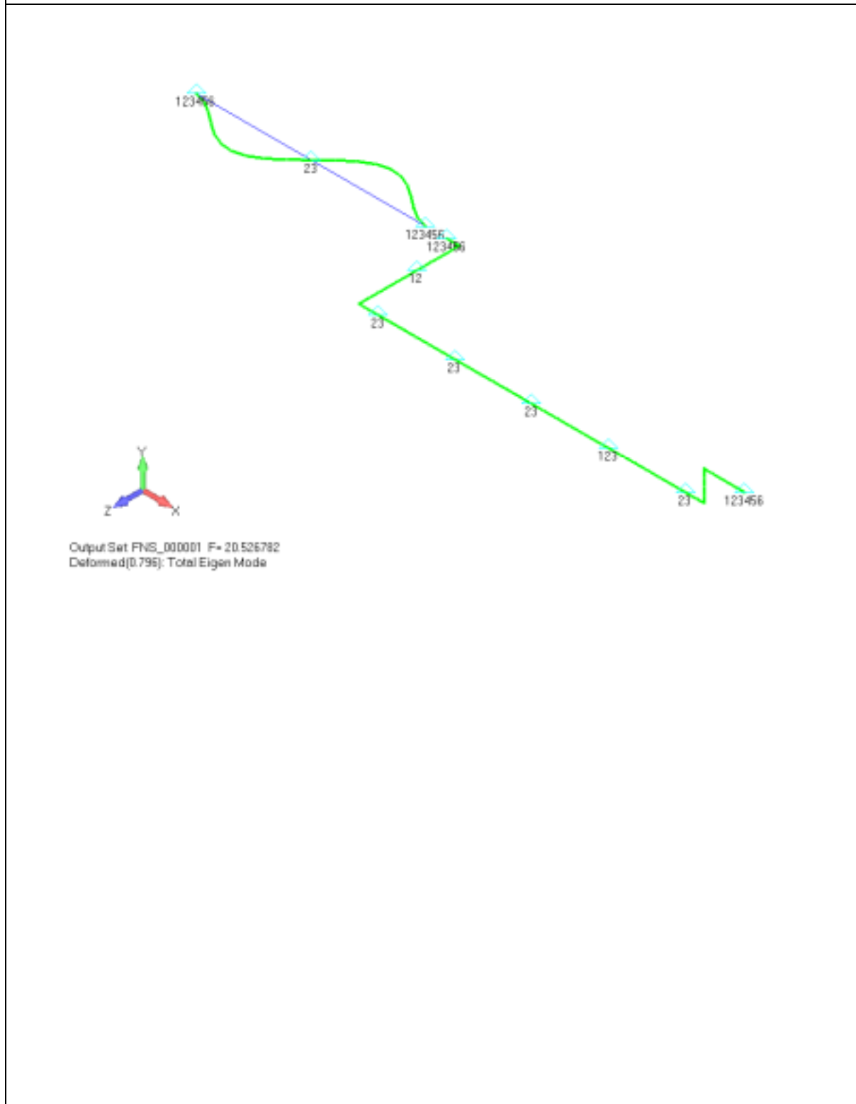
図 4-2 配管トレンチ (T21) 内配管 (外管) 固有モード図
