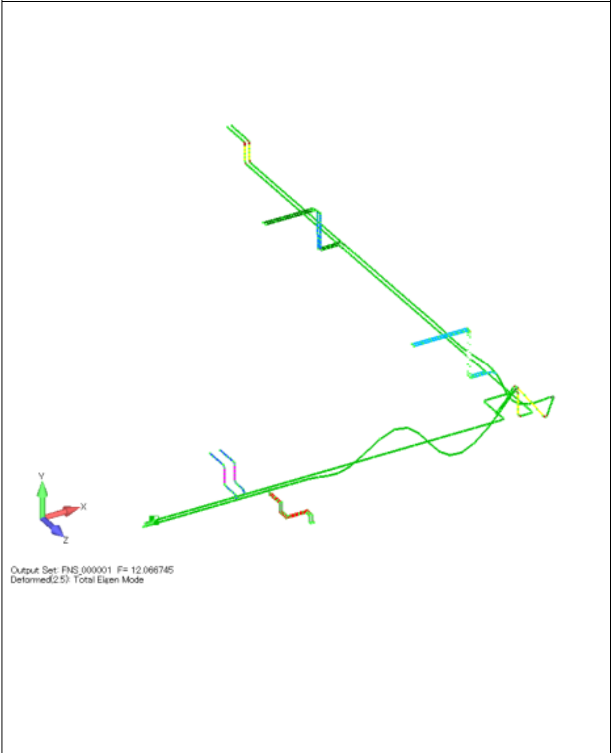
図 4-14-10 配管(KG84-617) 固有モード図 (1/3)
