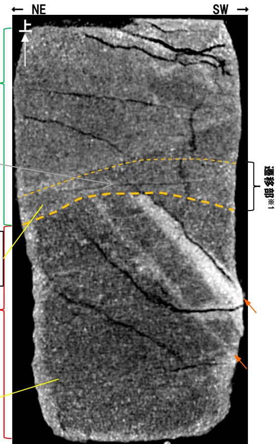
X線CT画像 (傾斜方向断面, 解釈線あり) (断面(B): 研磨片作成位置断面) 5cm
