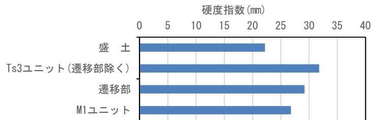
硬度測定結果(測線:SKB-a-2)
