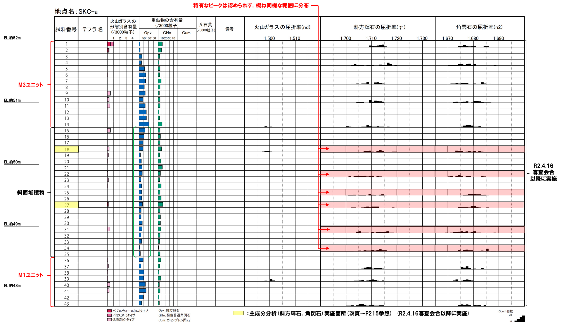
SKC-a 火山灰分析結果
