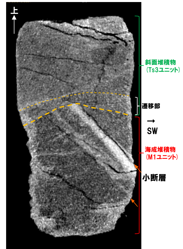
X線CT画像 (傾斜方向断面, 解釈線あり) (断面(A): 研磨片作成位置断面から手前方向に約5mmの位置)
