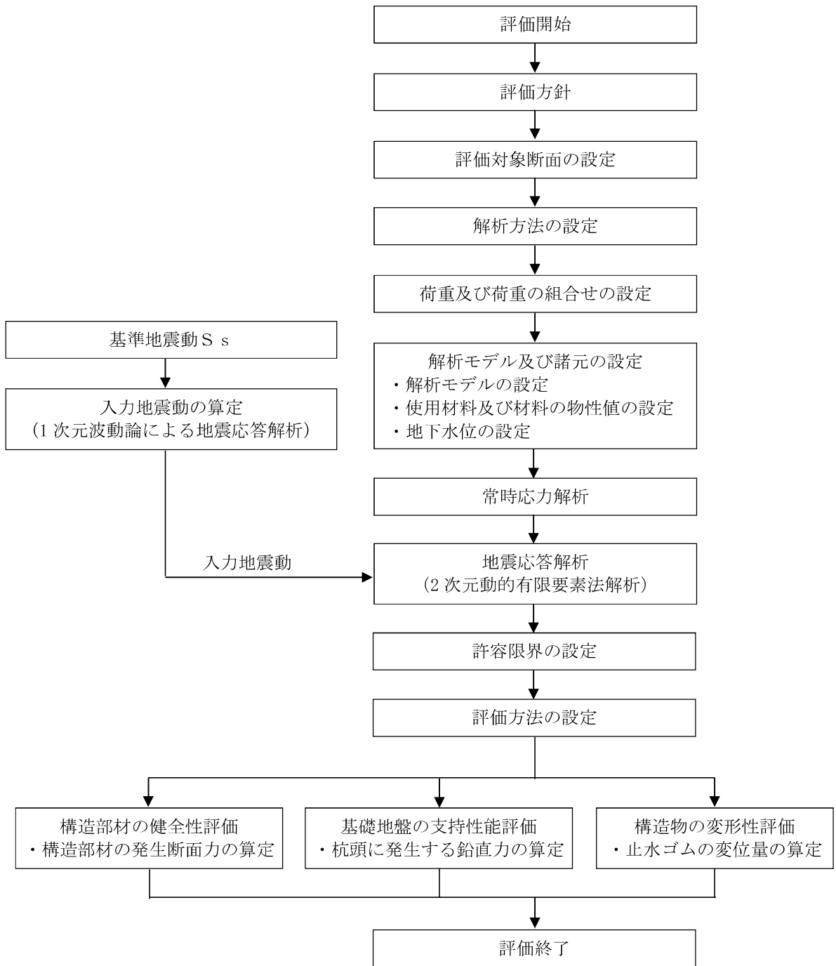
図 2-4 海水貯留堰（6号機設備）の耐震評価フロー
