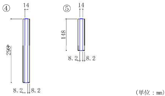
図 3-19 接合部の照査断面（照査断面寸法（溶接長）は腐食代を考慮）
