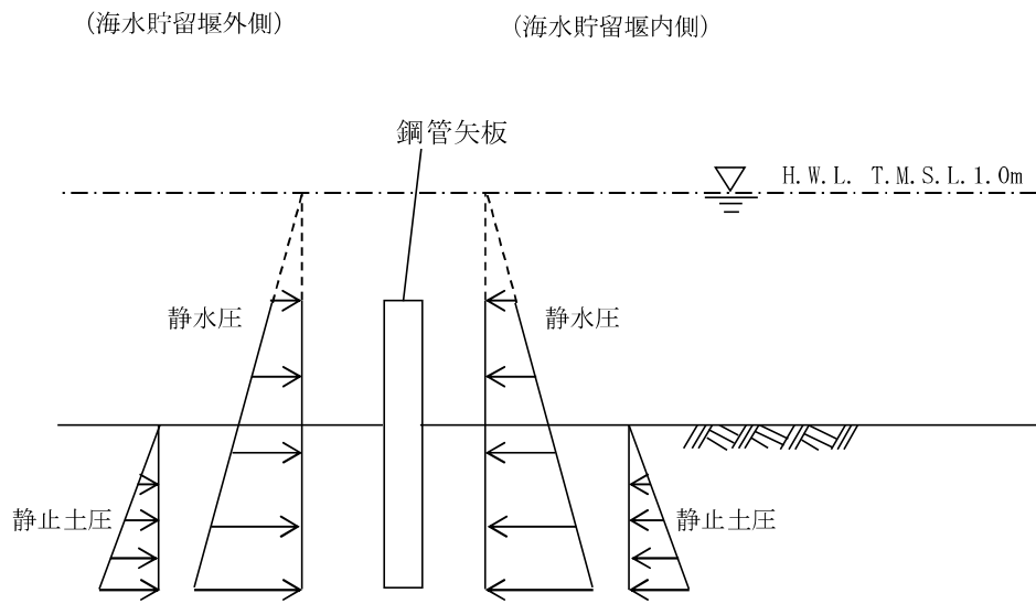
图 3-3 荷重作用图 (鋼管矢板 常時)
