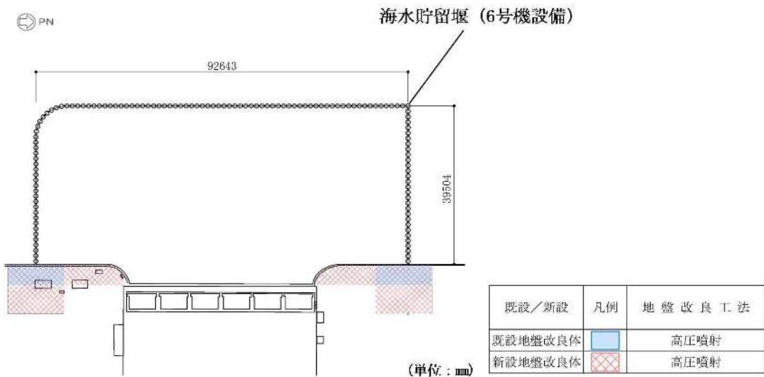
図2-1 (2) 海水貯留堰（6号機設備）の位置図（拡大図）
