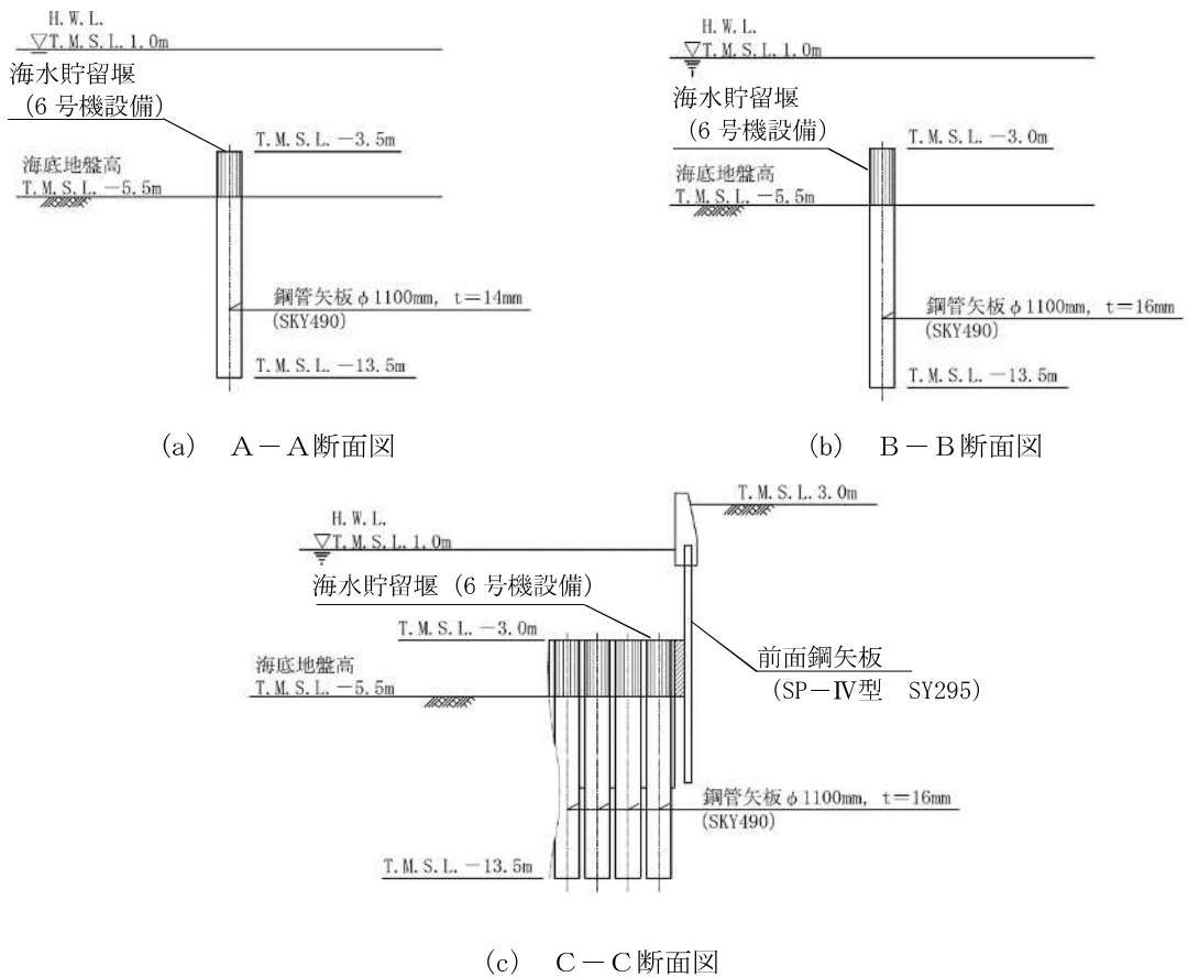
図 2-3 (1) 海水貯留堰 (6号機設備) の標準図
