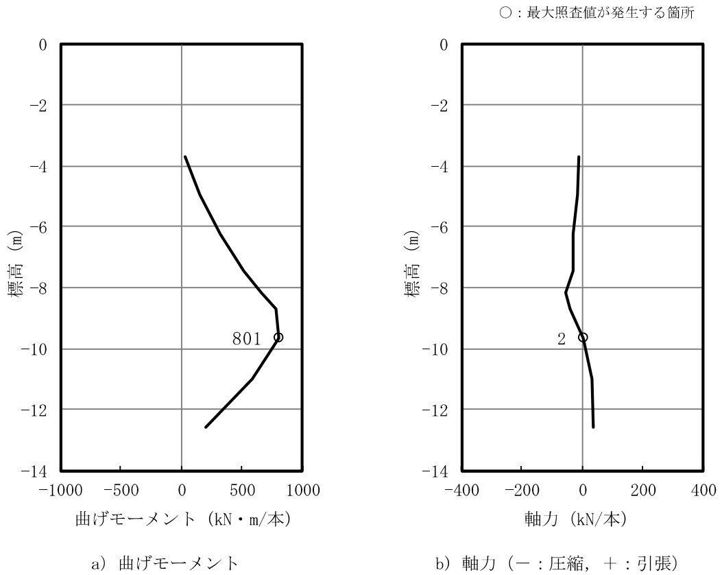
図3-9 (2) 鋼管矢板の曲げ軸力照査における最大照査値の評価時刻での断面力 (B-B断面 Ss-1++, t=5.87 s) (解析ケース③ : 地盤物性値のばらつき (-1σ) を考慮した解析ケース)
