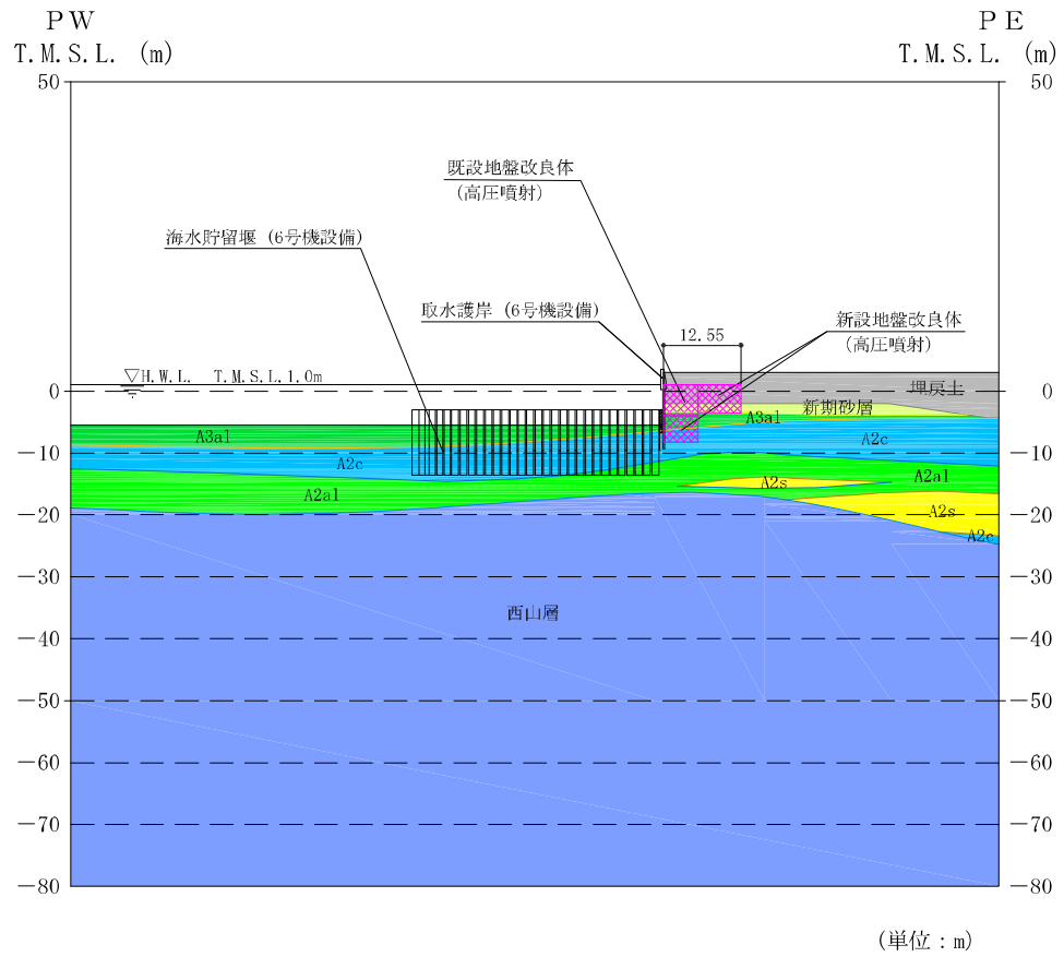
図 3-2 (1) 海水貯留堰 (6号機設備) の評価対象断面図 (A-A断面)
