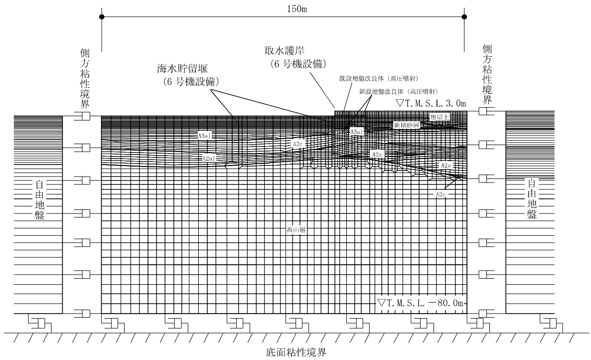
図 3-8 (1) 海水貯留堰 (6号機設備) の地震応答解析モデル (A-A断面)
