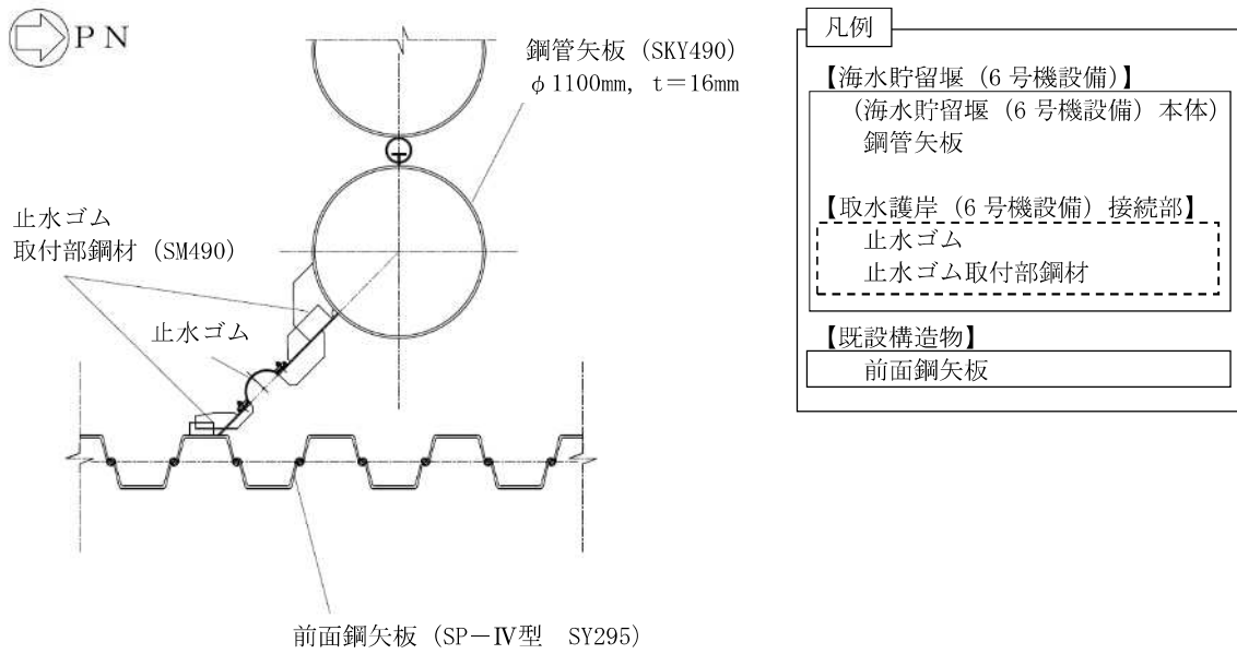
図 2-2 (2) 海水貯留堰 (6号機設備) の平面図 (A部拡大)
