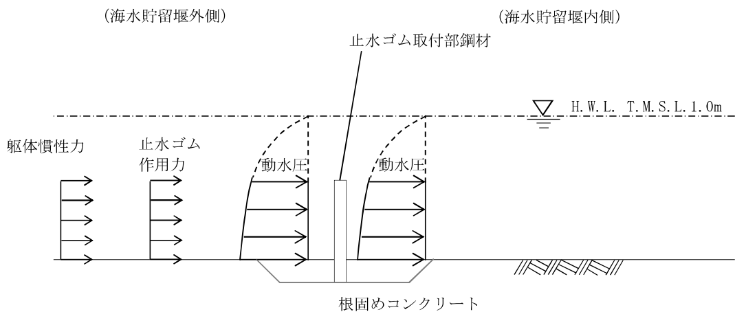
図 3-5 荷重作用図（止水ゴム取付部鋼材 地震時）
