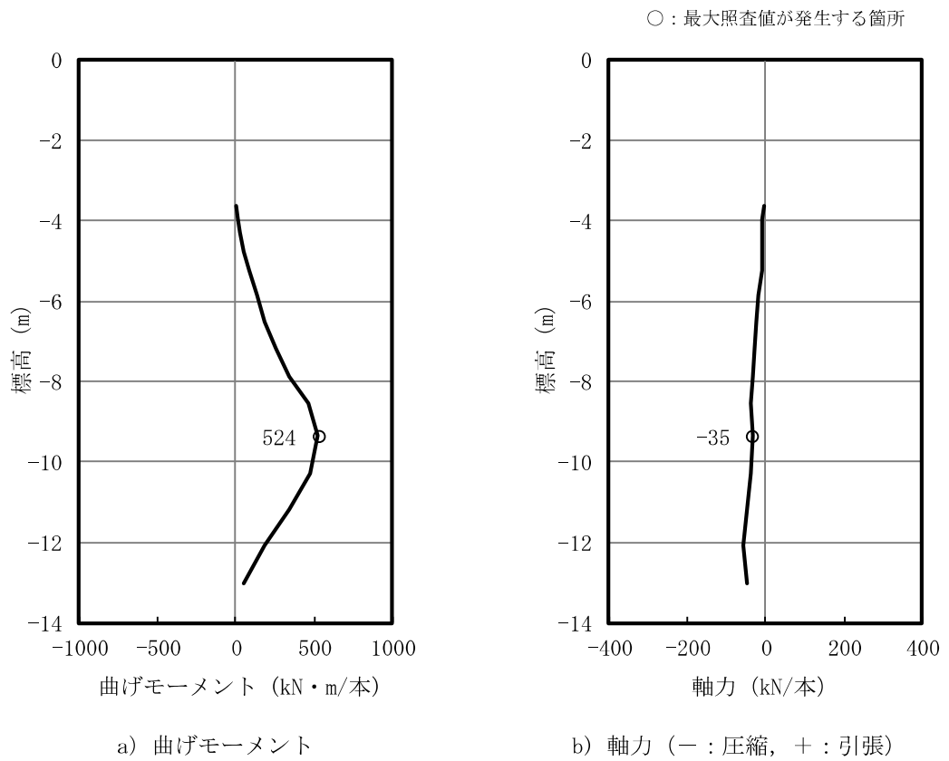
図3-9 (1) 鋼管矢板の曲げ軸力照査における最大照査値の評価時刻での断面力 (A-A断面 Ss-2EW, t=22.61 s) (解析ケース③ : 地盤物性値のばらつき (-1σ) を考慮した解析ケース)
