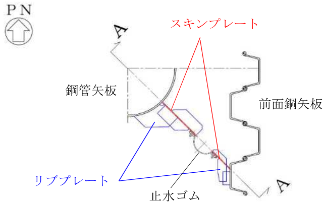
(a) 平面図
