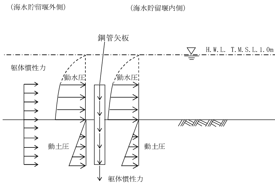
图 3-4 荷重作用图 (鋼管矢板 地震時)
