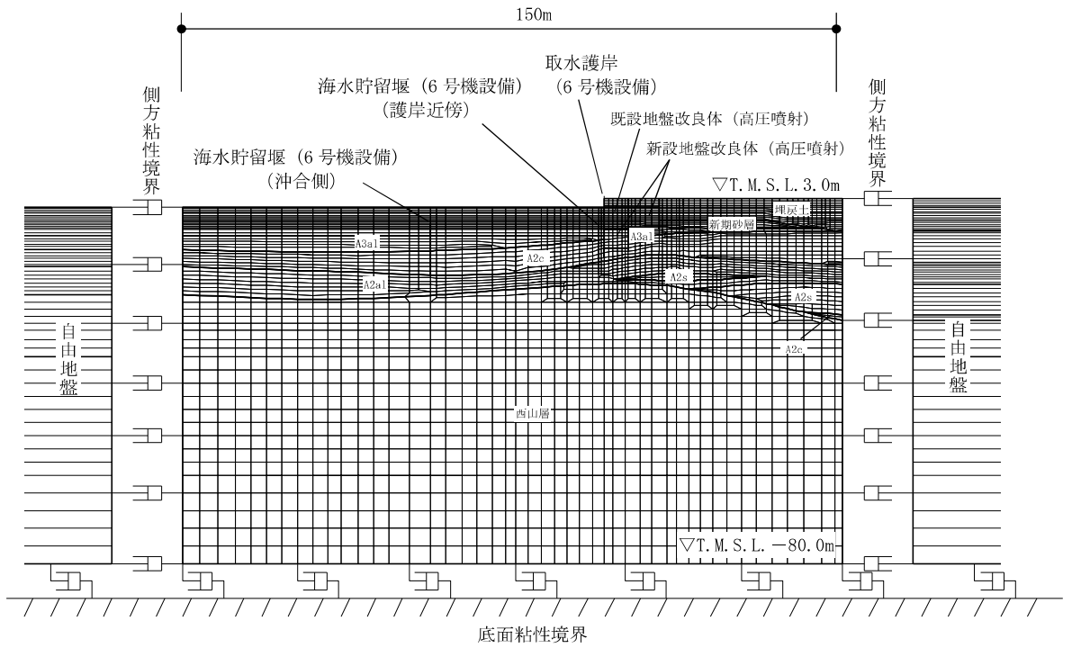
図 3-21 海水貯留堰 (6号機設備) の地震応答解析モデル
