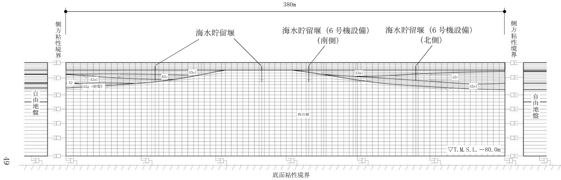
図3-8 (2) 海水貯留堰 (6号機設備) の地震応答解析モデル (B-B断面)
