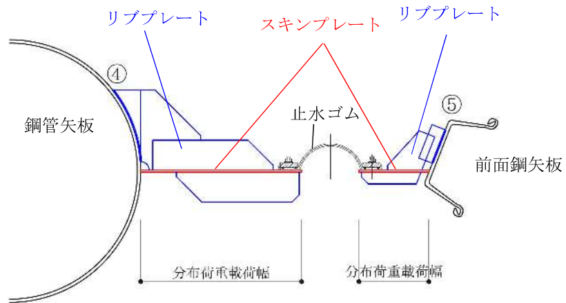
照査位置図
