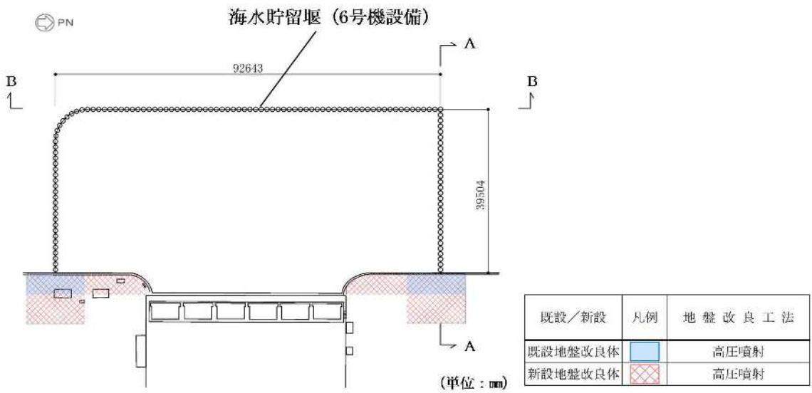
図3-1 海水貯留堰（6号機設備）の評価対象断面位置図
