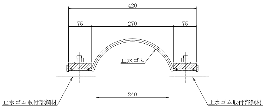
図 3-13 止水ゴムの構造図
