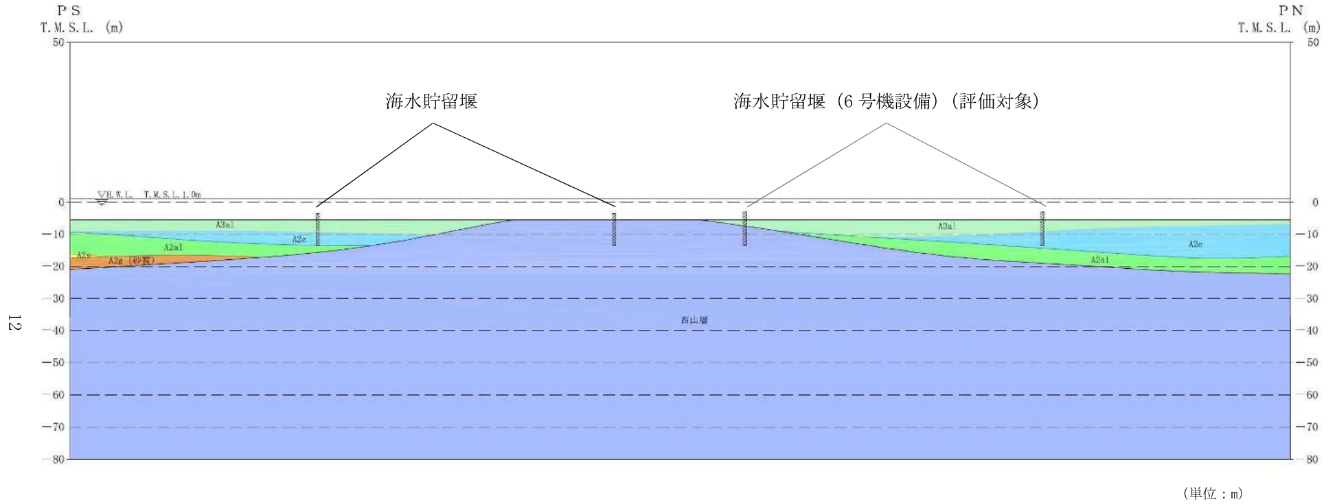
図 3-2 (2) 海水貯留堰 (6 号機設備) の評価対象断面図 (B-B 断面)
