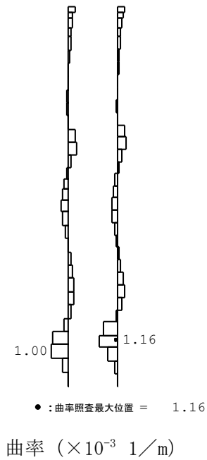
図 4-3 (1) 鋼管杭の曲げ軸力照査における最大照査値の評価時刻での曲率分布図 (A-A断面, Ss-1--, t=6.90s) (検討ケース③: 地盤物性のばらつき (-1 \sigma ) を考慮した解析ケース)
