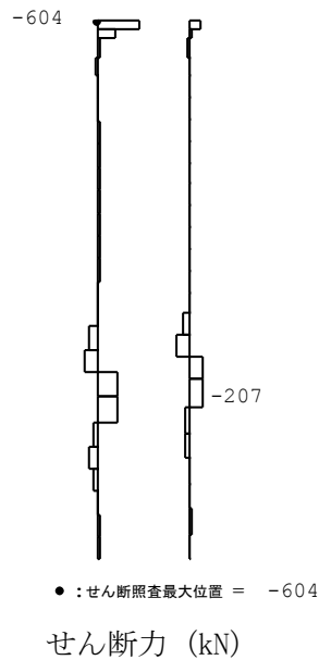
図 4-4 (2) 鋼管杭のせん断力照査における最大照査値の評価時刻での断面力 (杭一本あたり) (B-B断面, Ss-1++, t=6.77s) (検討ケース③: 地盤物性のばらつき (-1 \sigma ) を考慮した解析ケース)
