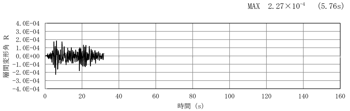
図 4-1 (1) 鉄筋コンクリート部材の曲げ軸力照査における層間変形角の時刻歴波形 (A-A断面, Ss-1+-) (検討ケース①: 基本ケース)
