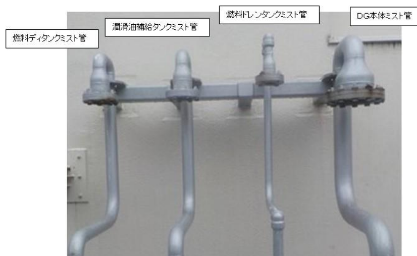
図6-9 ミスト管
