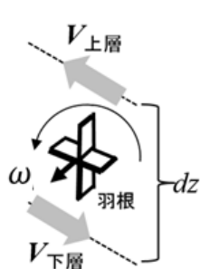
水平渦度生成に関する模式図
