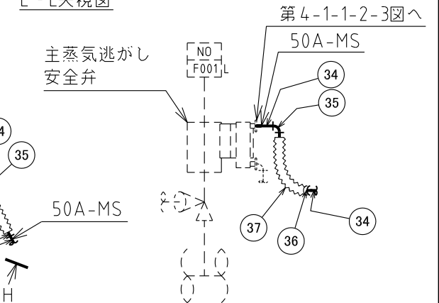
G部詳細図
