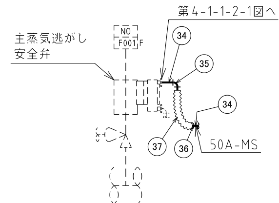
G部詳細図
