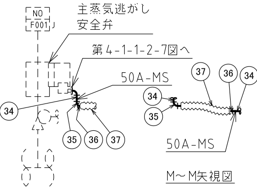
L~L矢視図
