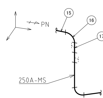
A~A矢視図
