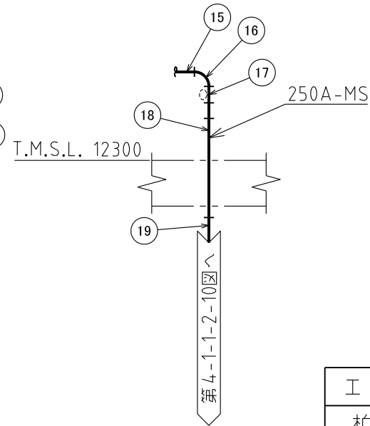
H~H矢視図
