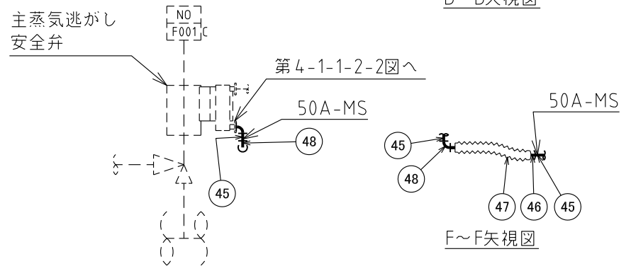
E~E矢視図
