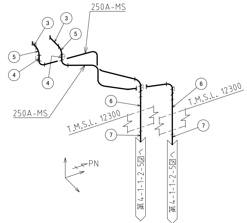
C部詳細図
