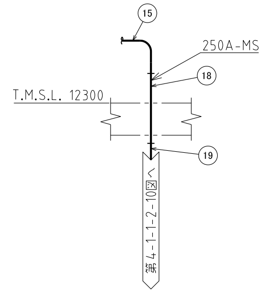
E~E矢視図
