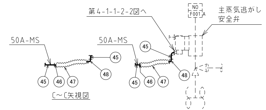
D~D矢視図
