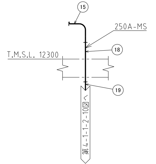
F~F矢視図
