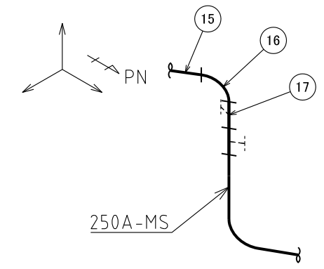
B~B矢視図
