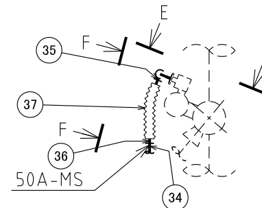
D部詳細図
