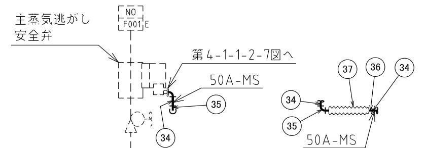
F部詳細図
