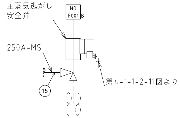
A~A矢視図
