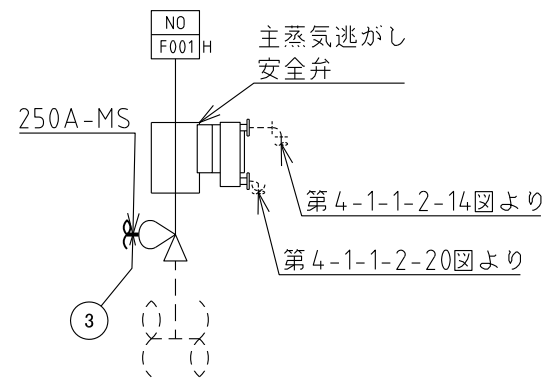
C~C矢視図
