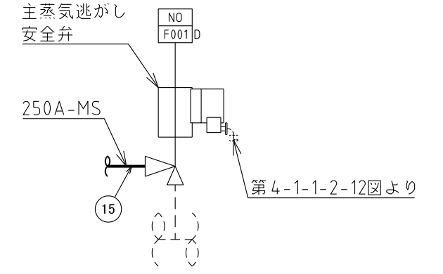
B~B矢視図
