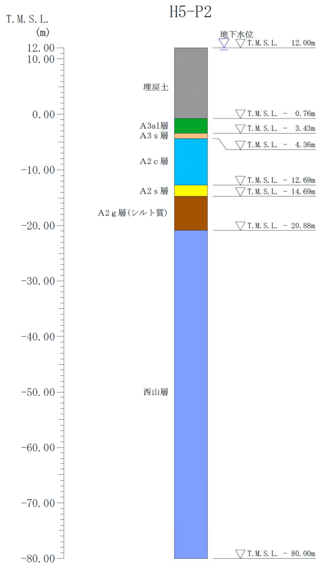
図 2-13 1次元地震応答解析モデル (可搬型重大事故等対処設備保管場所 (5号機東側保管場所))
