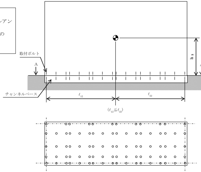
A~A矢視図
