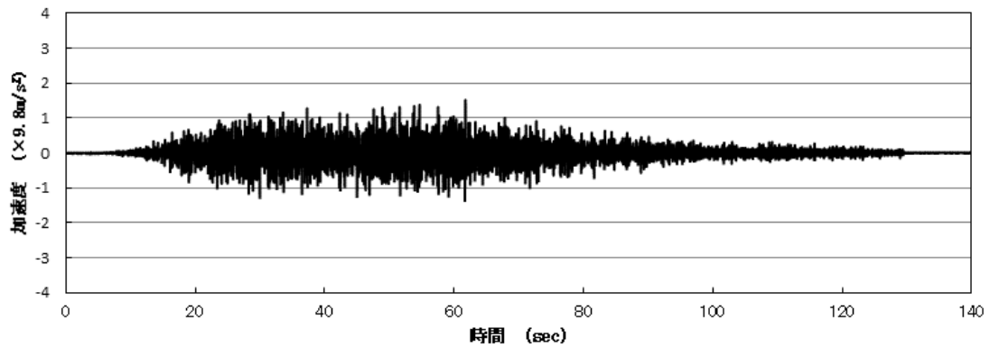
図 3-1 加振試験に用いた加振波の加速度時刻歴 (試験体 A) (フラップゲート開, 水なし)
