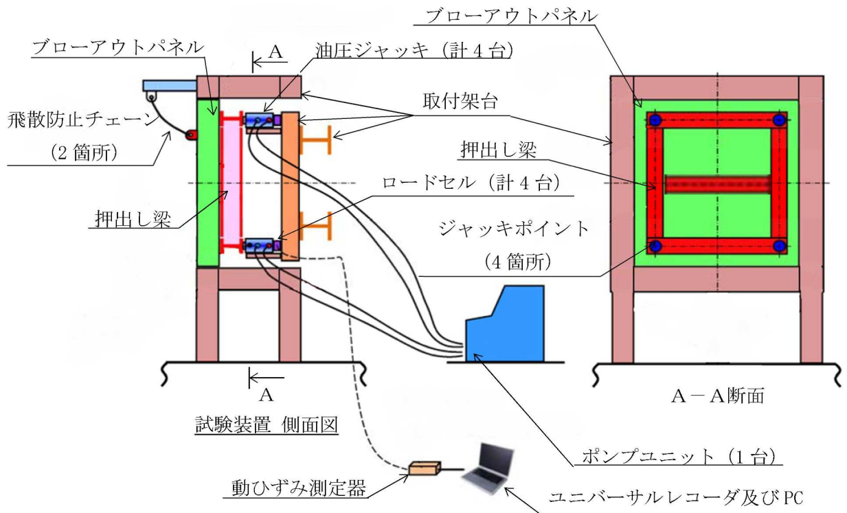
図6-1 オペフロBOP実機大モックアップ試験装置の概要
