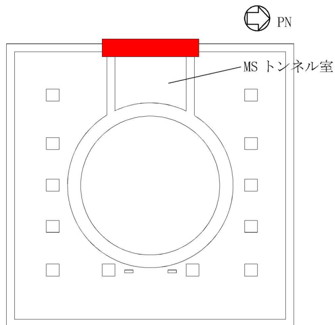
原子炉建屋原子炉区域地上1階 概略平面図
