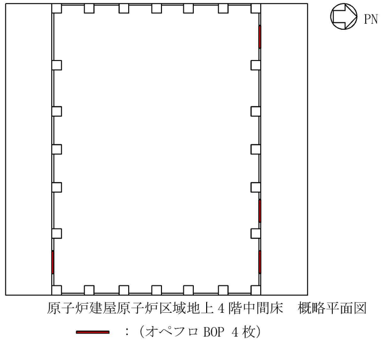
図7-1 オペフロ BOP の設置位置
