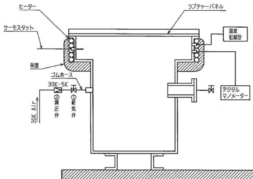
図6-2 破裂試験装置の概要（断面図）
