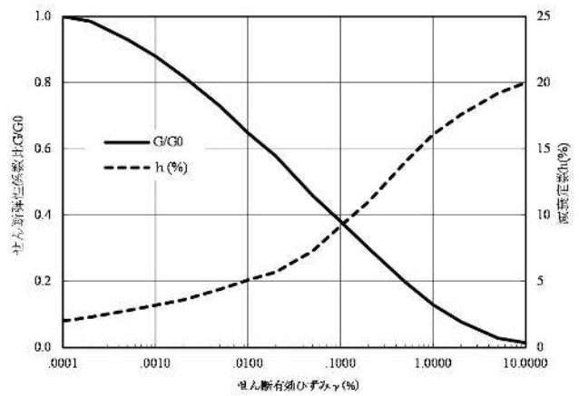
図 3-5 ひずみ依存特性(第 1 層)
