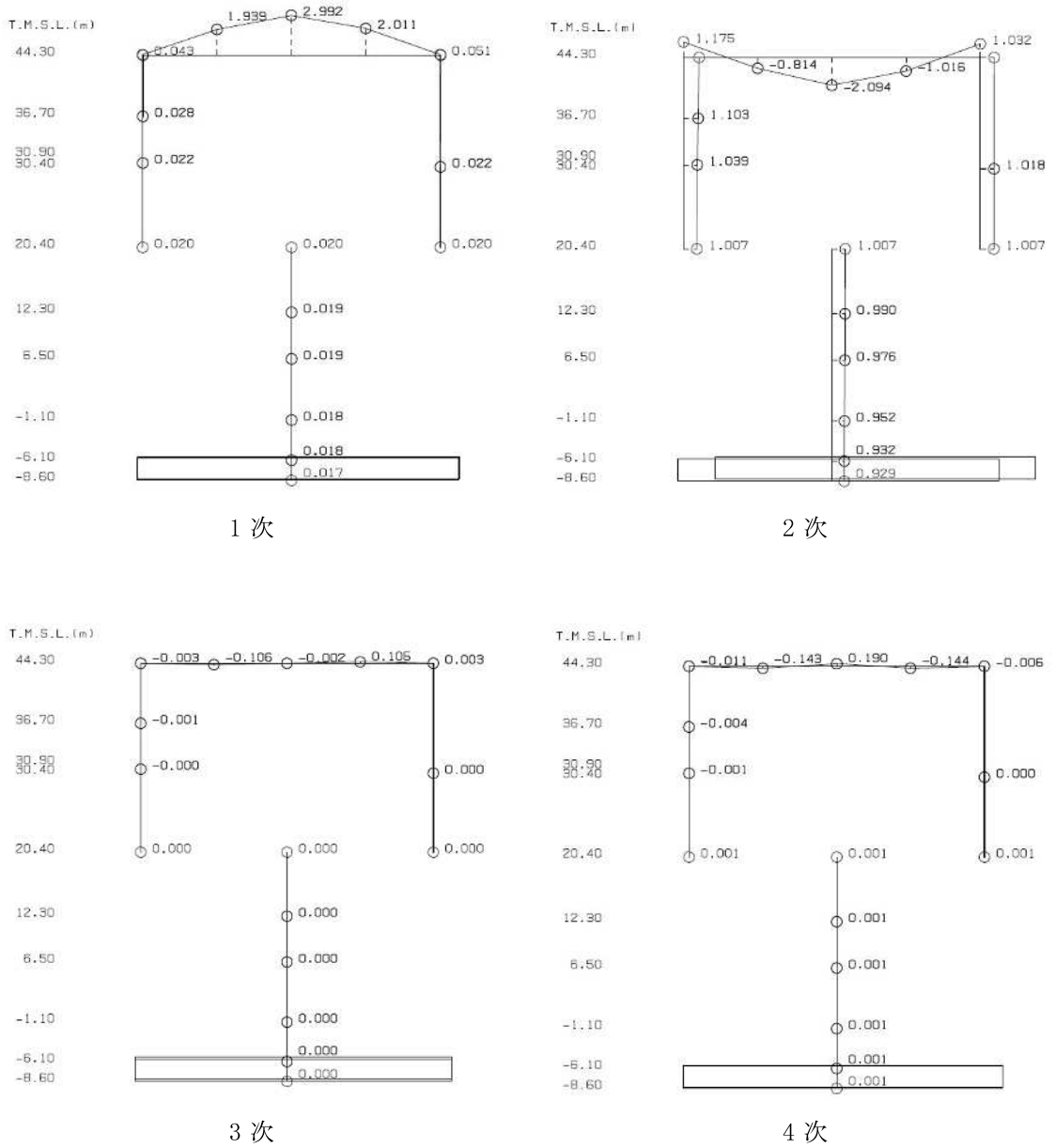
図 4-1 刺激関数図 (Ss-1, 鉛直方向) (3/3)
