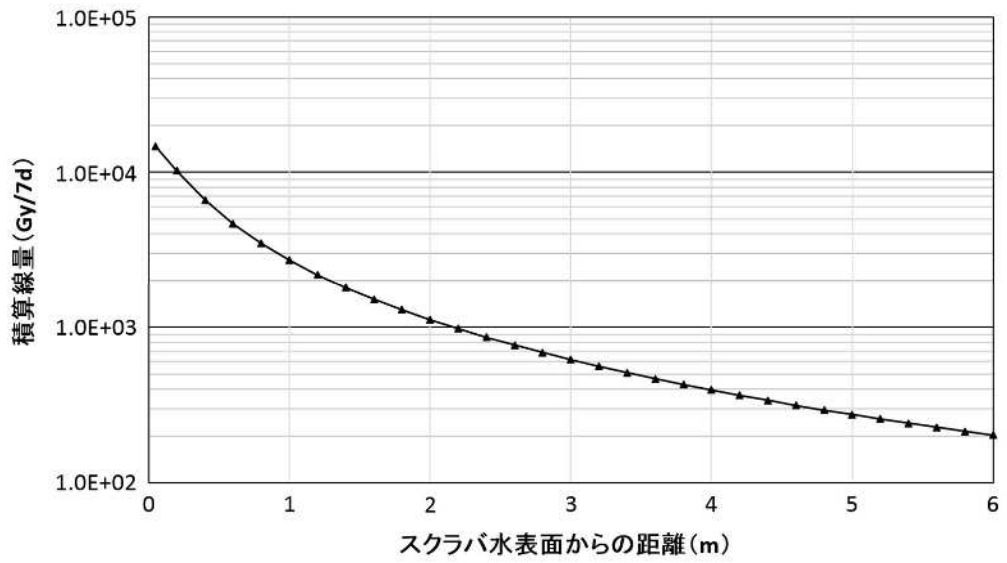
図4 スクラバ水からの距離と線量
