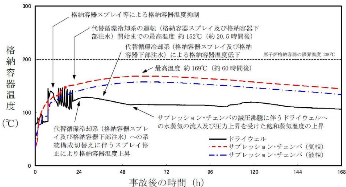
図 3 「高圧溶融物放出/格納容器雰囲気直接加熱等」におけるサブプレッションチェンバ(気相)温度時刻歴
