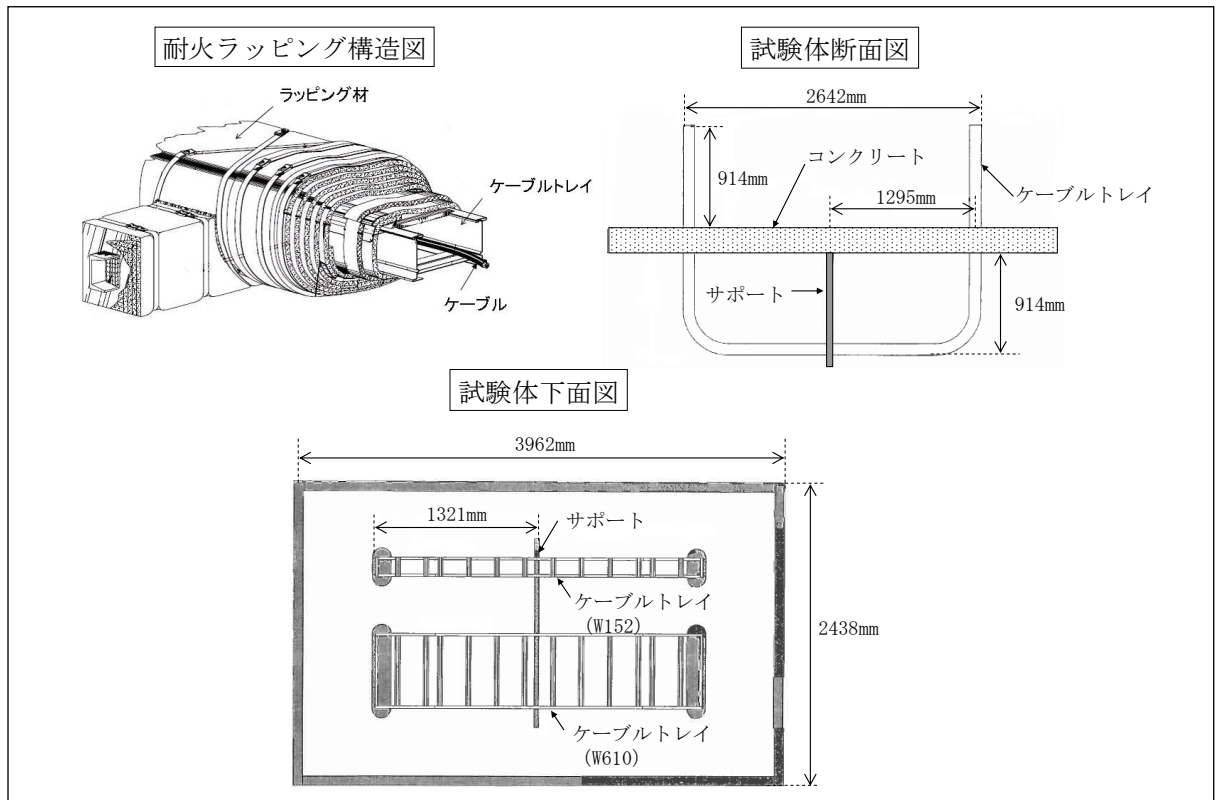
図 6-8 耐火ラッピングの耐火試験体
