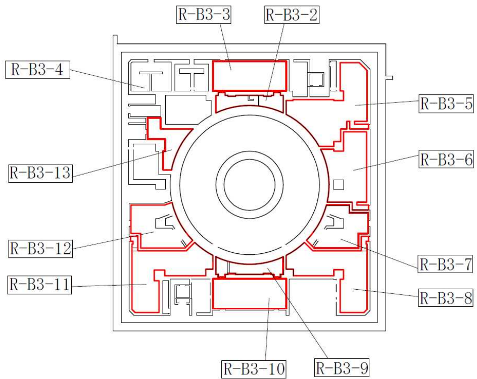
原子炉建屋 T. M. S. L. -8200
