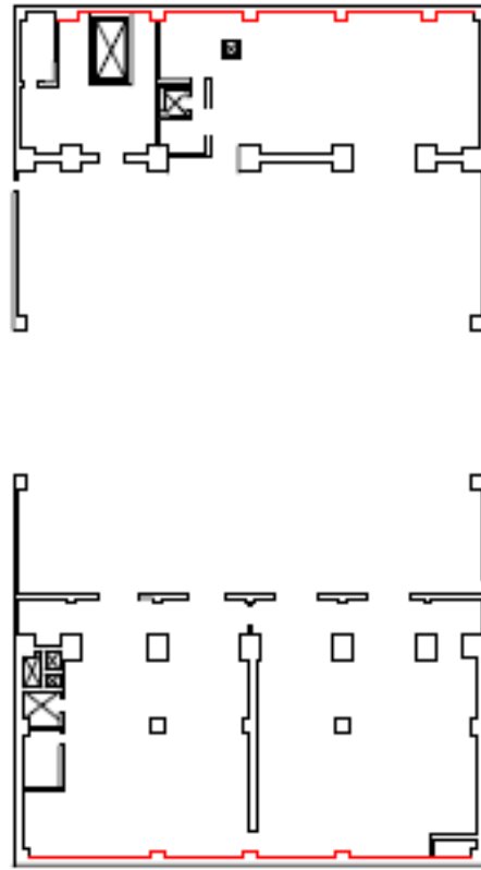
廃棄物処理建屋 T. M. S. L. 20400
