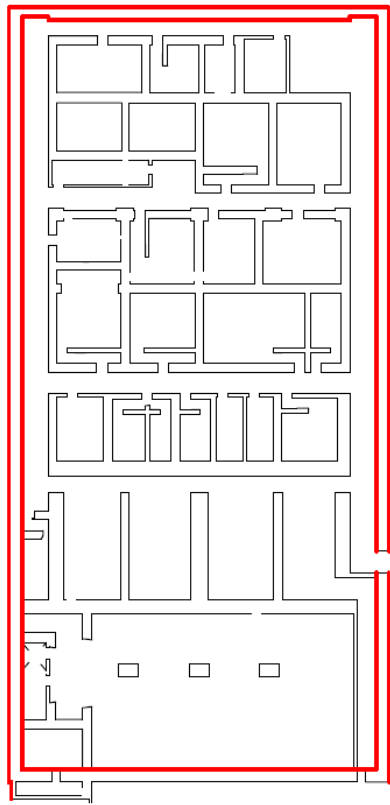
廃棄物処理建屋 T.M.S.L. -6100
