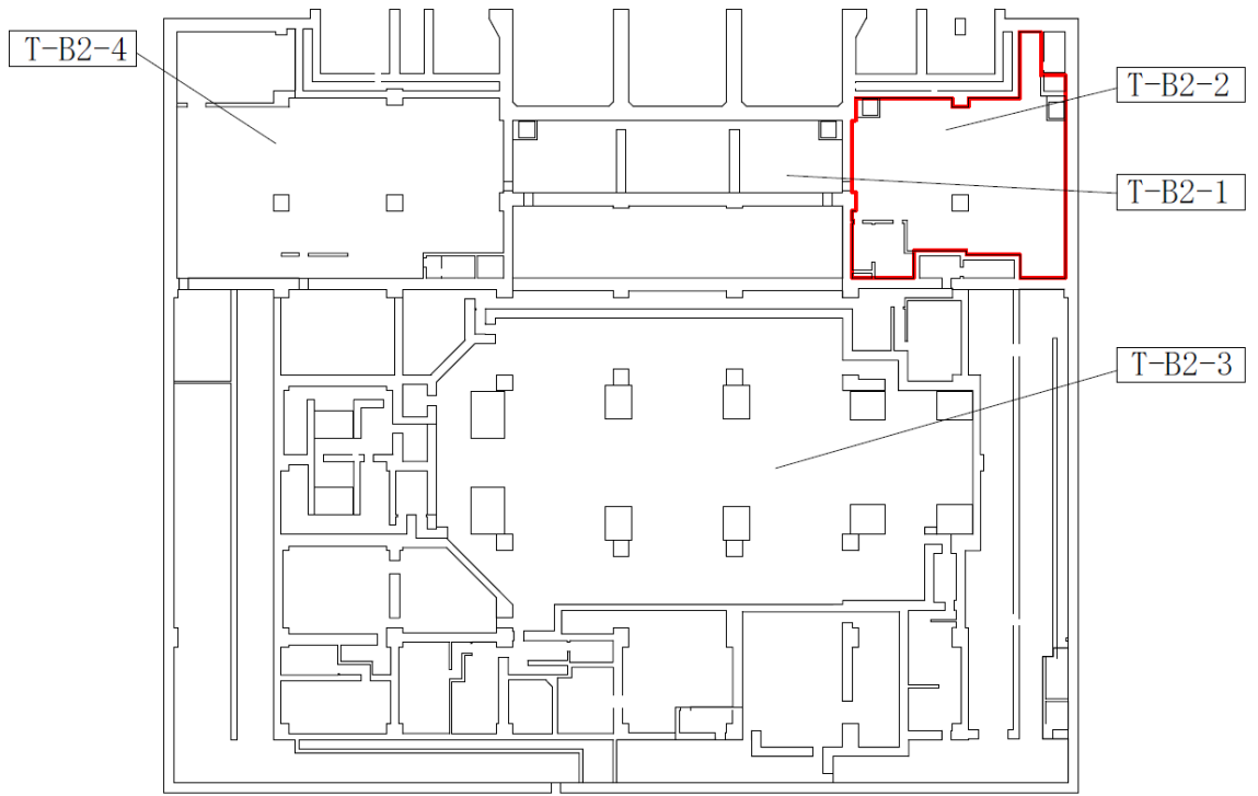
タービン建屋 T.M.S.L. -5100
