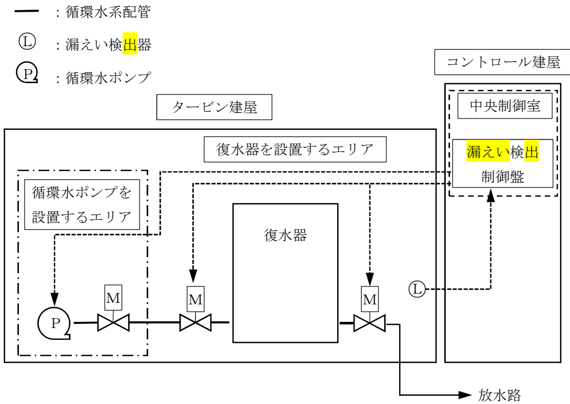
第 4-12 図 循環水系隔離システムの概要
