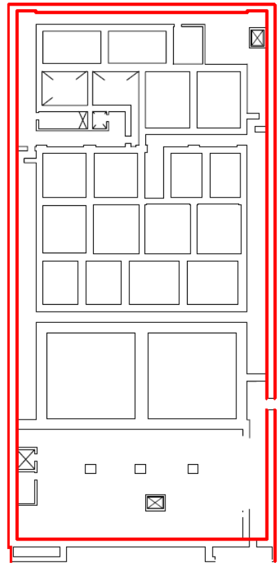
廃棄物処理建屋 T.M.S.L. -1100
