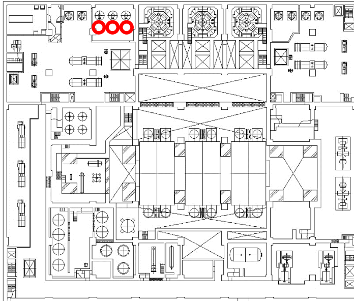
タービン建屋 T. M. S. L. 4900
