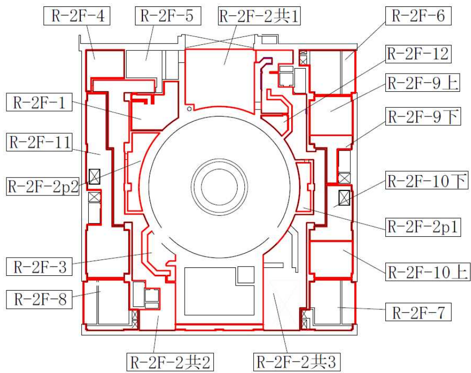
原子炉建屋 T. M. S. L. +18100
