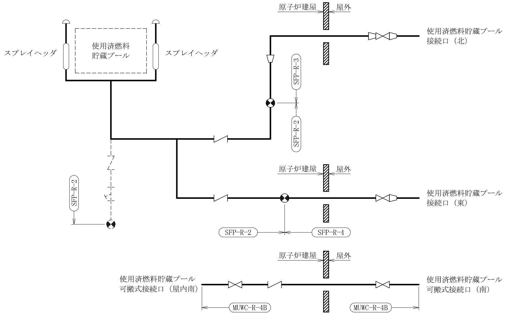
燃料プール代替注水系概略系統図
