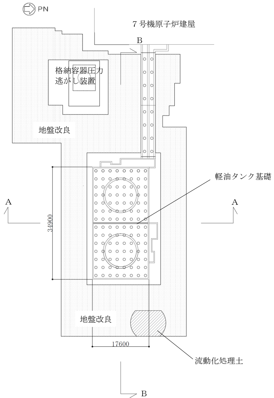
図 2-2 軽油タンク基礎の平面図
