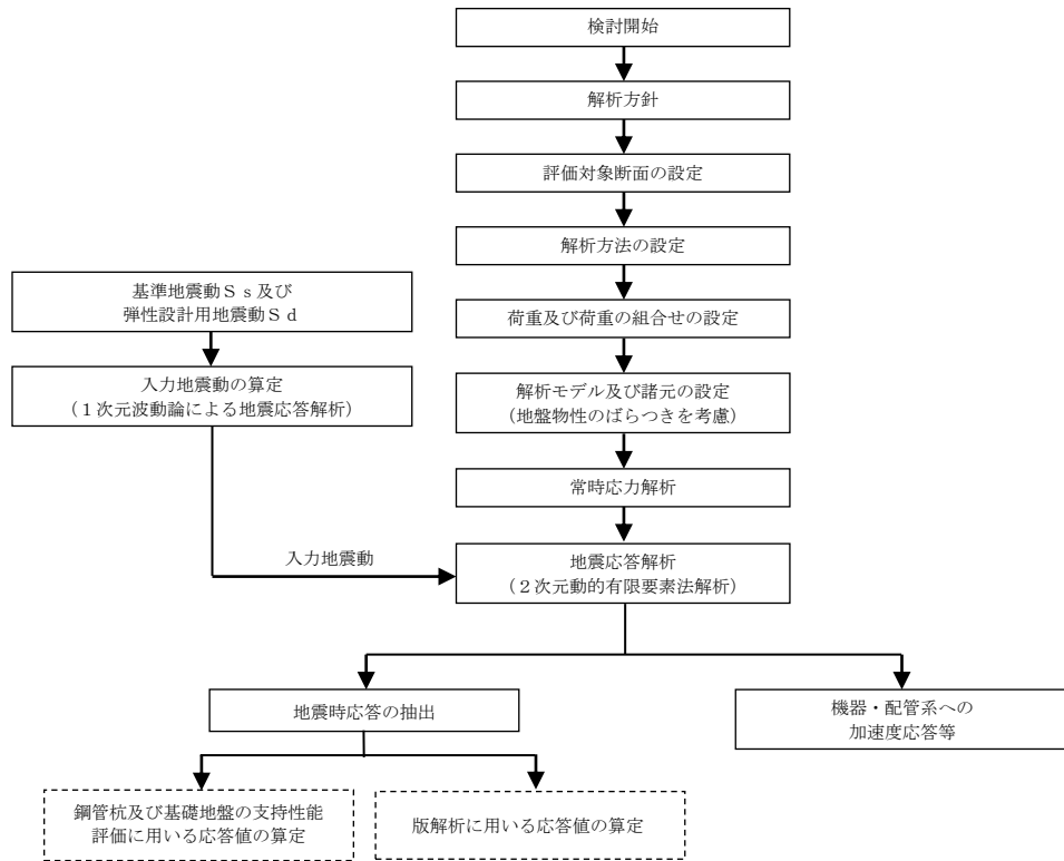
図 2-4 軽油タンク基礎の地震応答解析フロー
