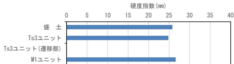
硬度測定結果(測線:SKB-TW⑦)
