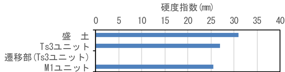
硬度測定結果 (測線:SKB-FF③)
