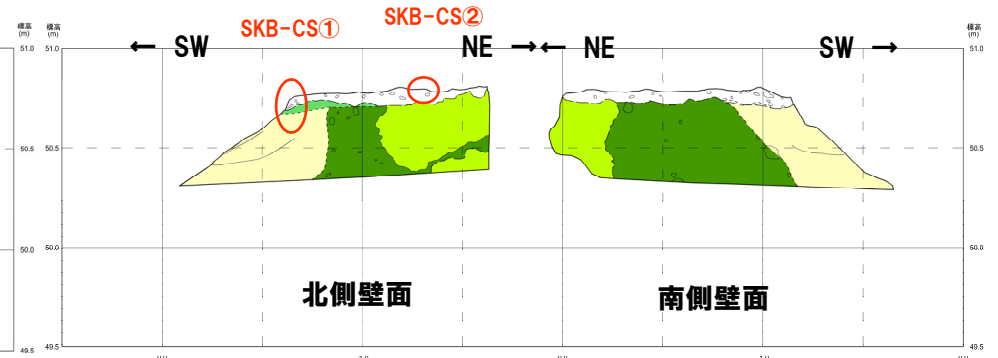
開削調査箇所(南側)横断掘削箇所③ スケッチ
