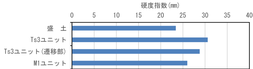
硬度測定結果(測線:SKB-TW①)
