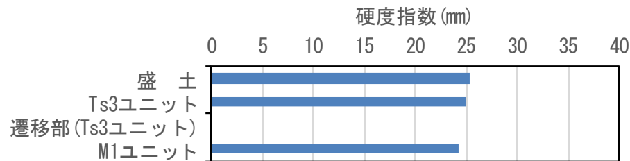
硬度測定結果 (測線:SKB-FF⑤)
