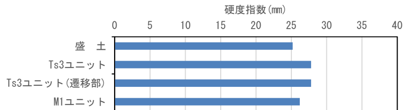
硬度測定結果(測線:SKB-TW⑤)
