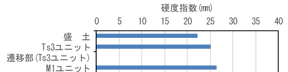
硬度測定結果 (測線:SKB-FF④)
