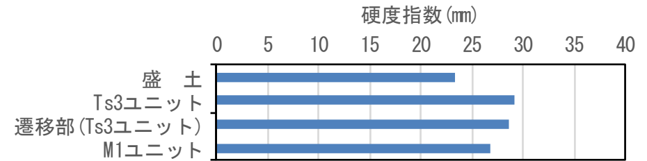
硬度測定結果 (測線:SKB-FF②)
