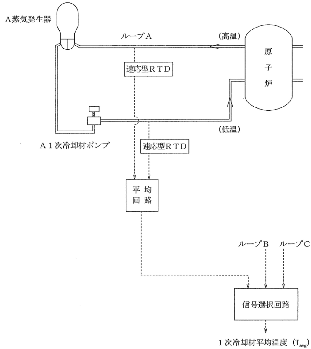
第1.7-2図 1次冷却材平均温度測定説明図
