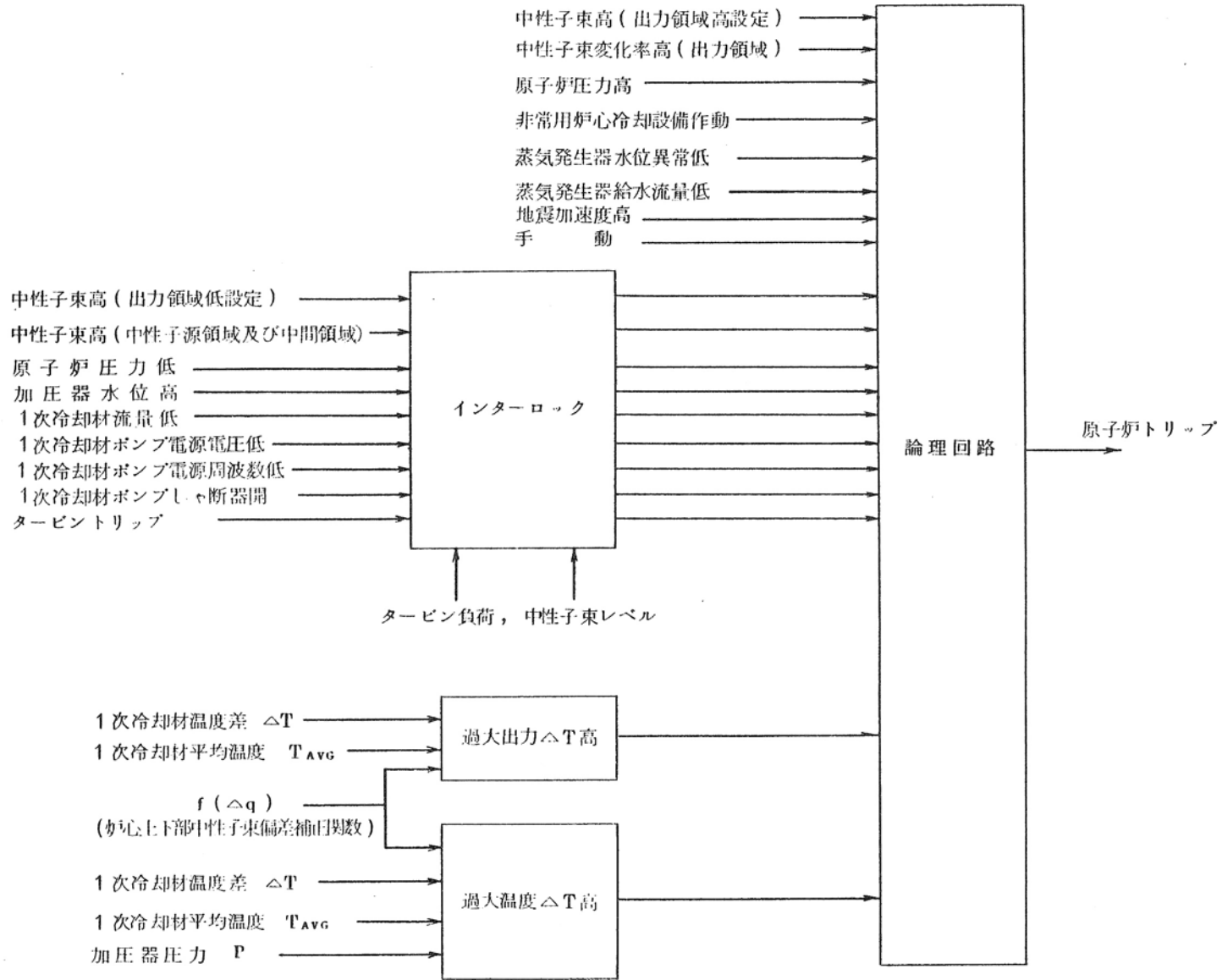
第1.7-8図 原子炉保護系説明図
