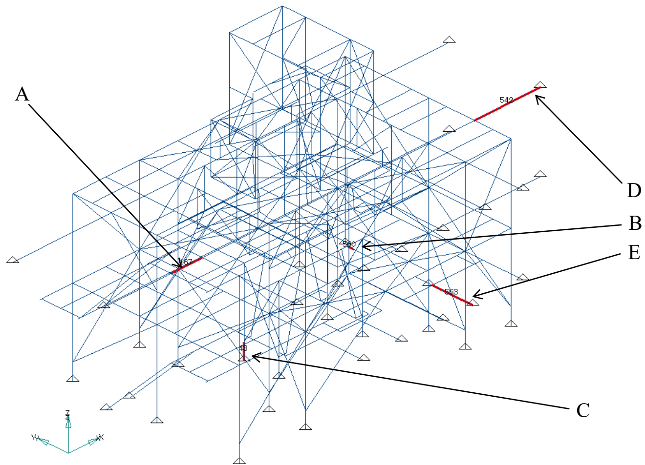
图 5-1(1/2) 实验装置架台 最大应力发生位置
