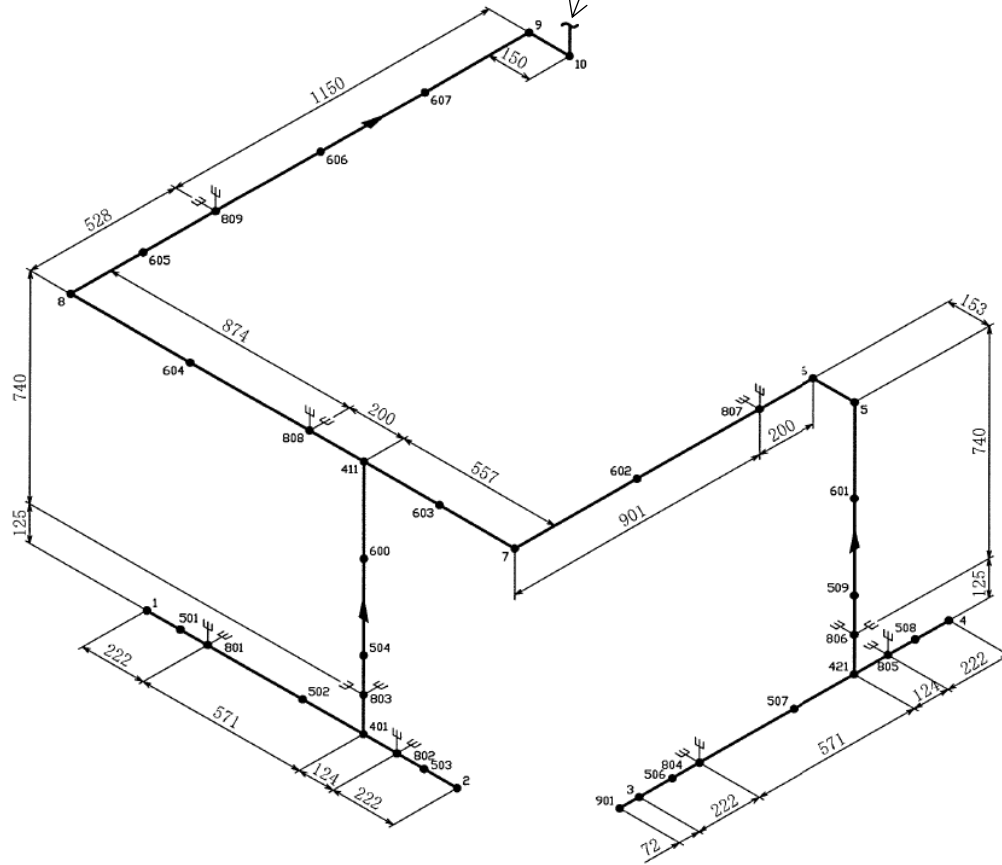
鳥瞰図 中央制御室床下フリーアクセスフロア (1/13)
