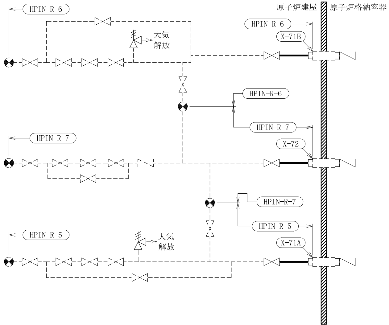
高压窒素ガス供給系概略系統図
