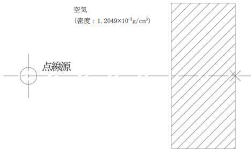
断面 A-A
