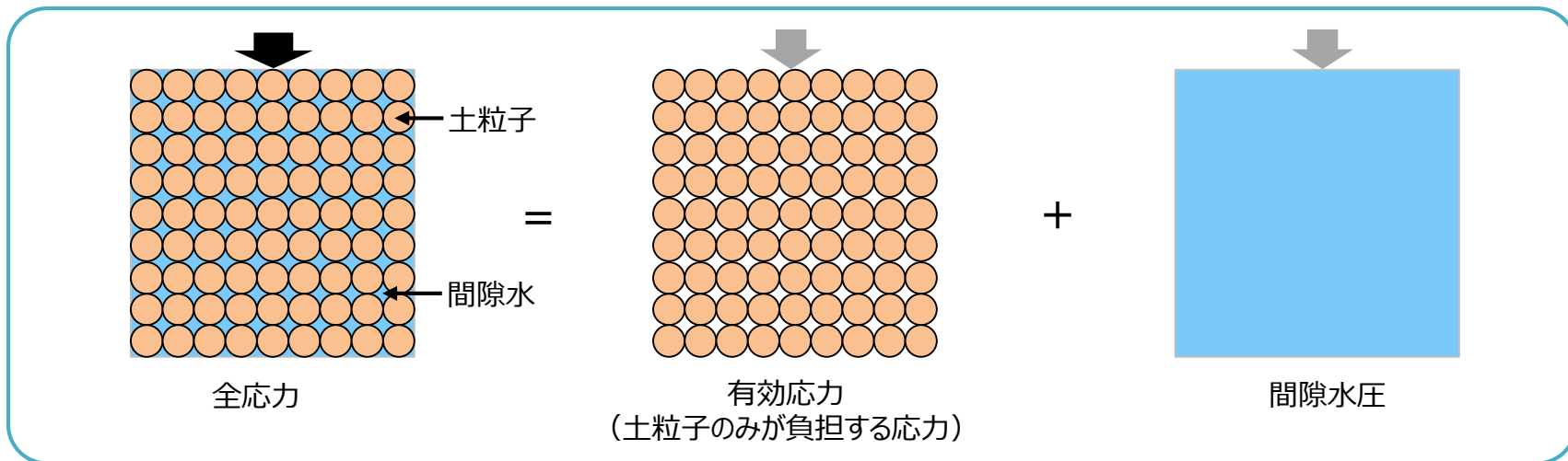
地盤の強度の概要
