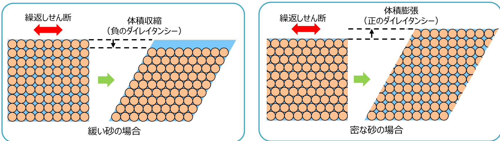
地盤のダイレイタンス特性の概要
