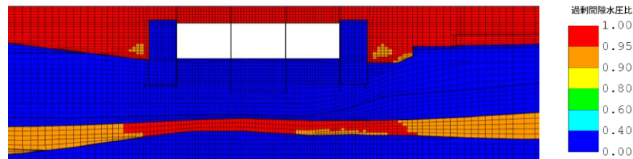
6号機取水路（漸縮部）の最大過剰間隙水圧比分布図 (解析ケース③, Ss-3--)
