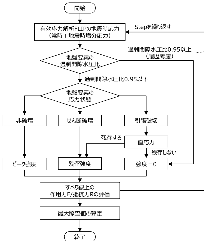
地震時の水平力・鉛直力に対する支持性能評価における照査値の算定フロー
