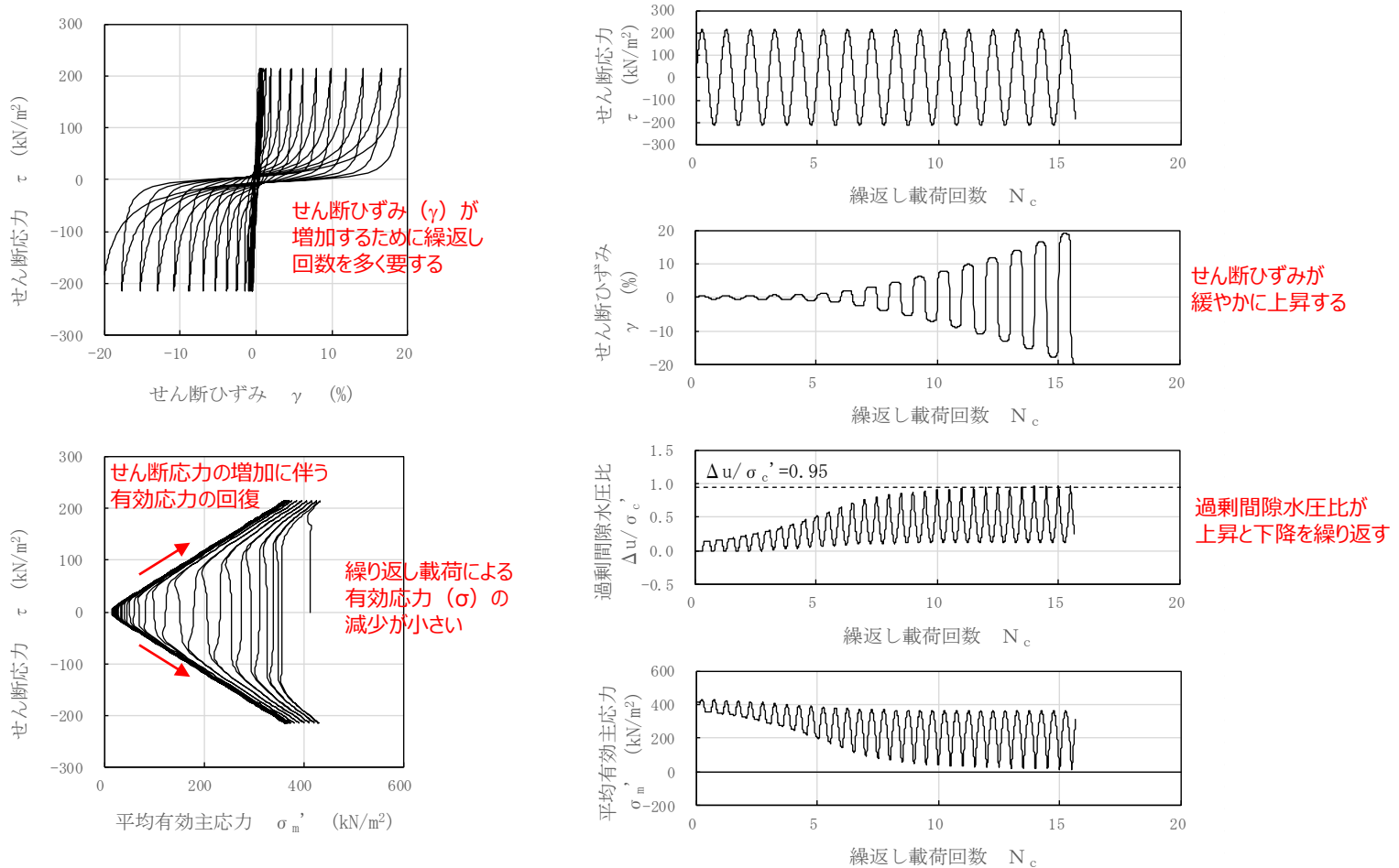
A2s層の要素シミュレーションの結果 (有効拘束圧412kN/m 2 , せん断応力比 R_{L20}=0.519 )
