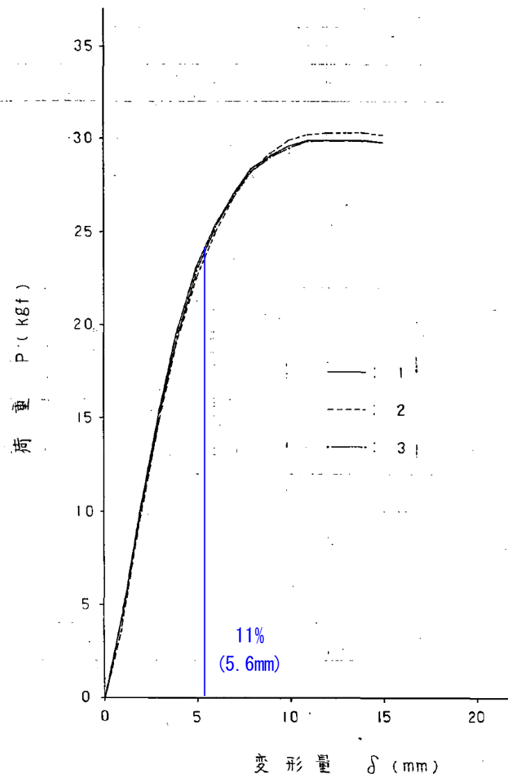
図 3-2 サブドレン管の荷重-変位曲線図
