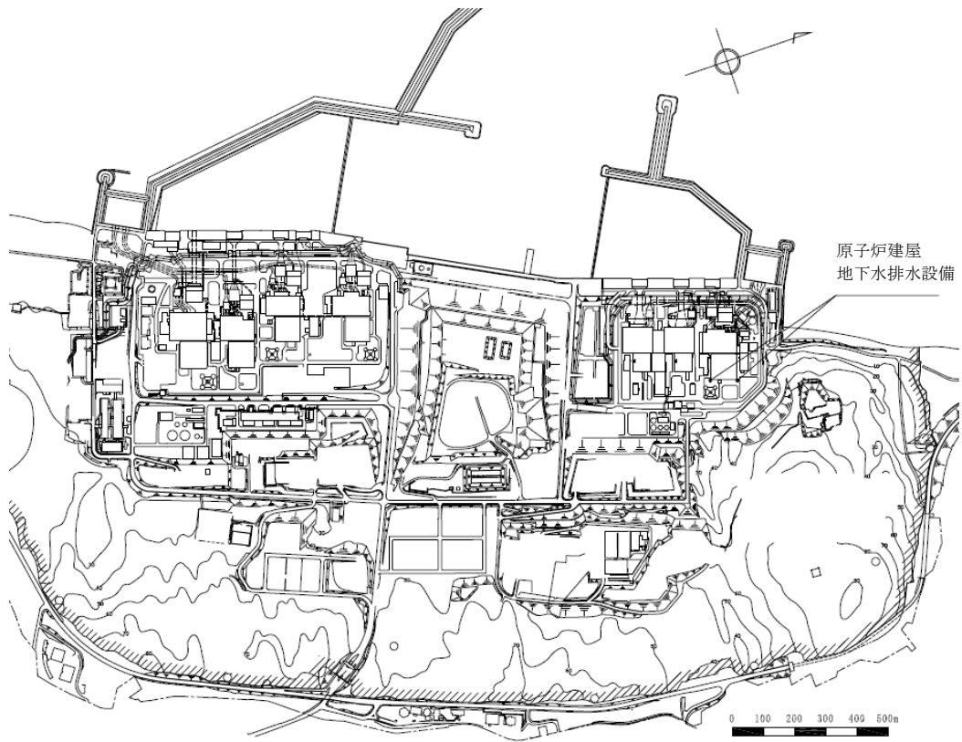
図 2-1 地下水排水設備の概略配置図
