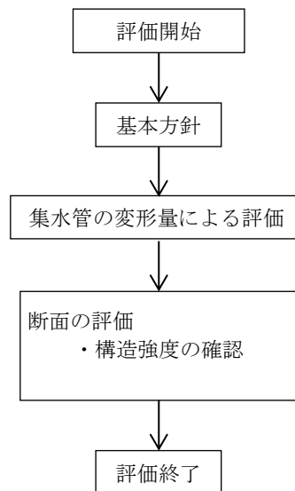
図2-3 集水管の評価フロー
