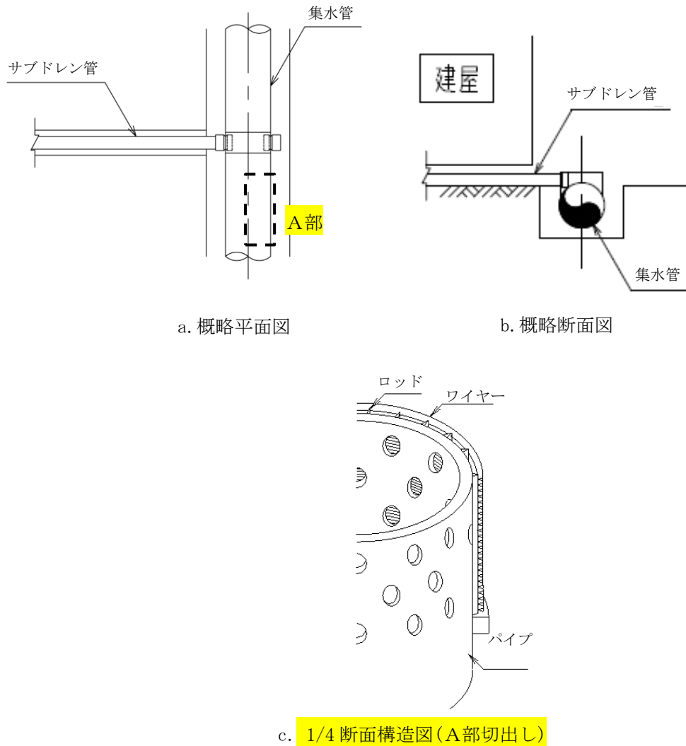
図2-2 概略平面図・断面図及び断面構造図
