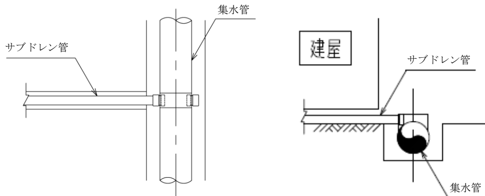
図2-2 概略平面図・断面図
