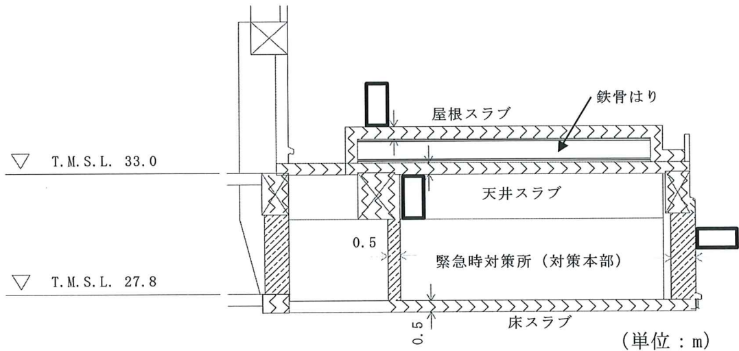
B-B 断面
