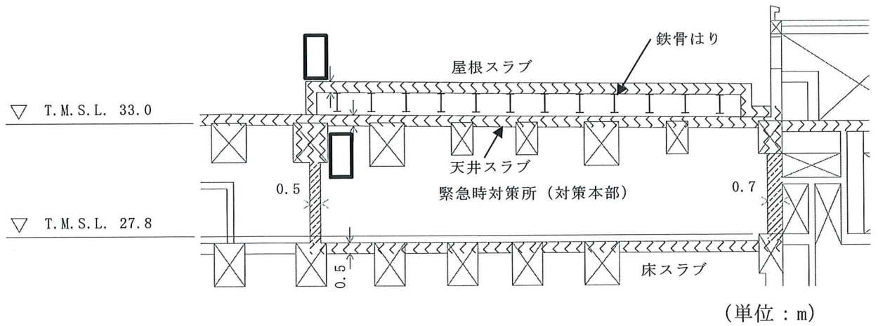
A-A 断面
