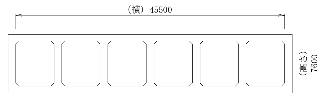
断面B~B
