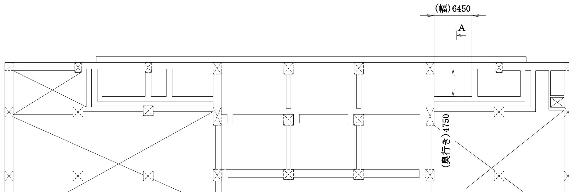
平面図
