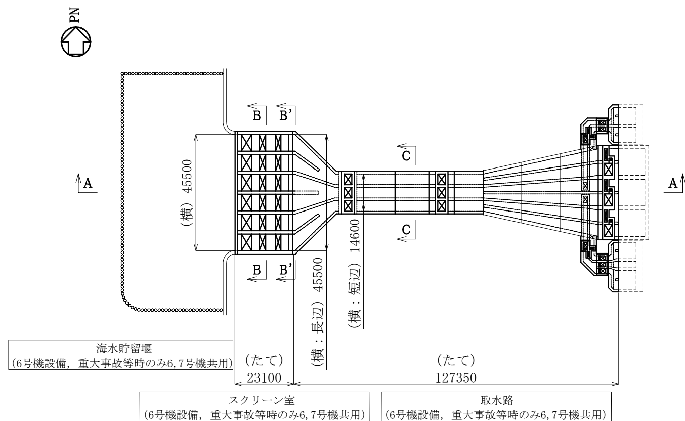
平面図
