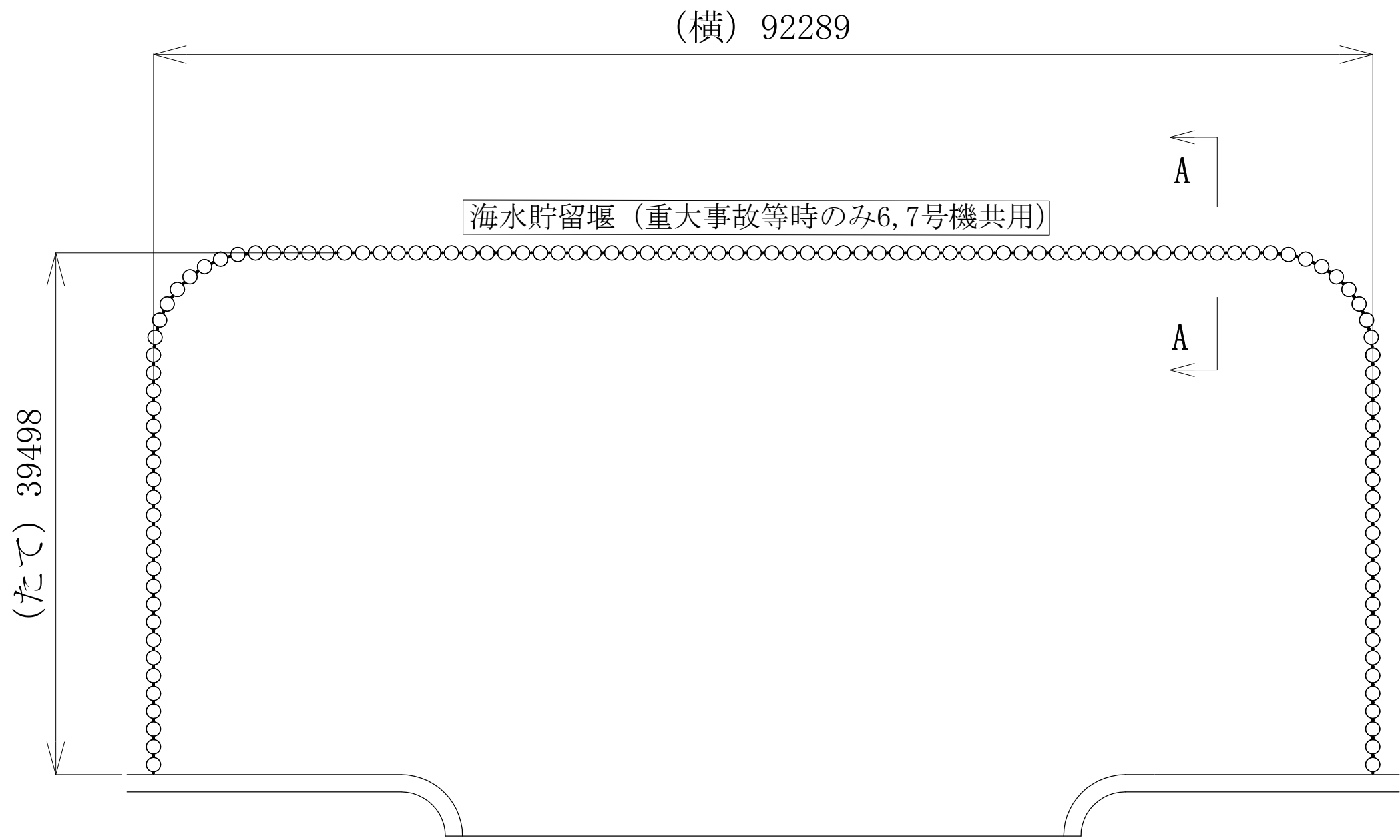
平面図
