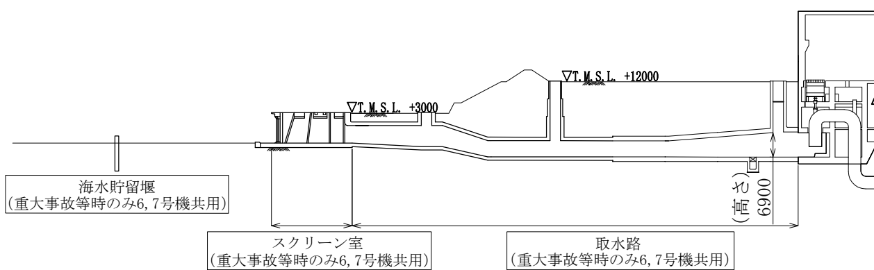
断面A~A
