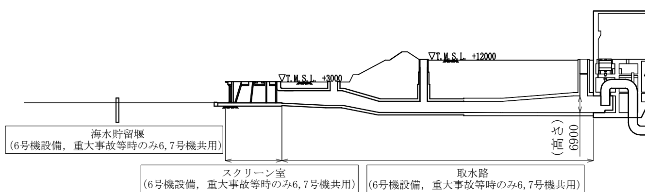
断面A~A
