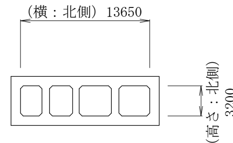
断面D~D
