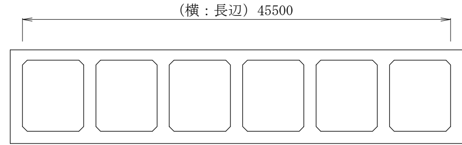
断面B'~B'
