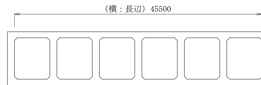
断面B'~B'
