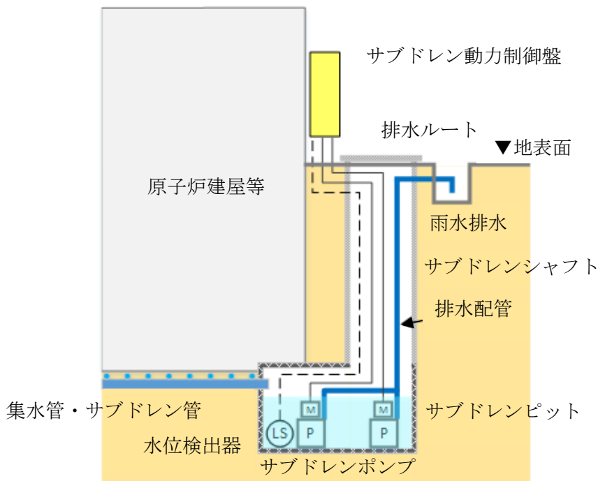
図1 7号機地下水排水設備の概要図
