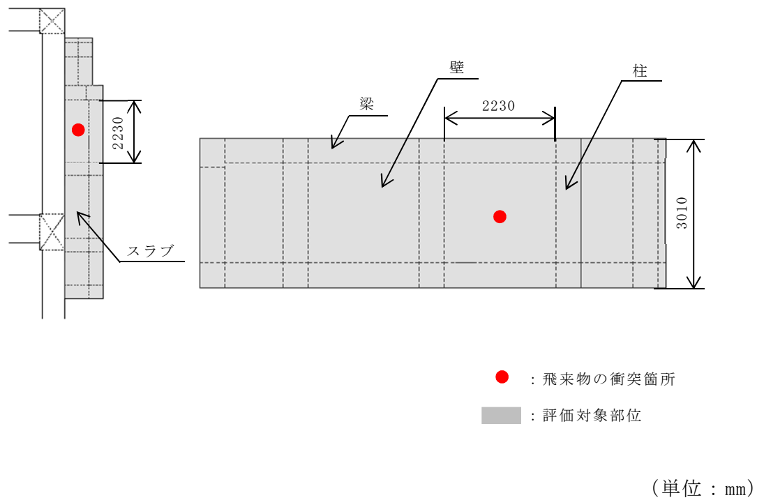
図 3-1 コンクリ製フードの評価位置図
