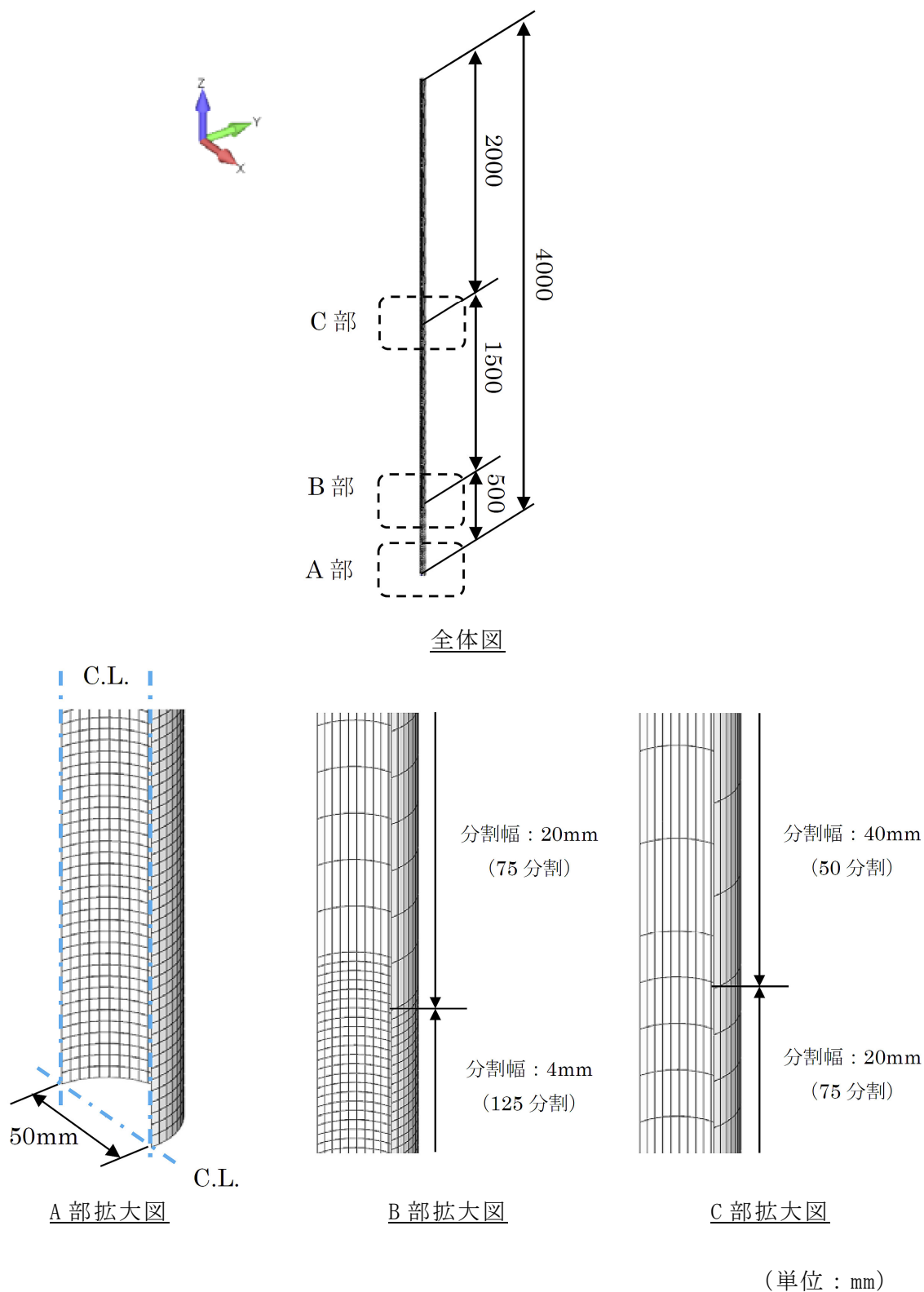
図 3-4 飛来物の解析モデル図 (足場パイプ 1/2 モデル)
