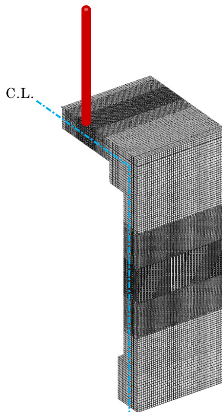
図 4-2 解析ケース（スラブ）
