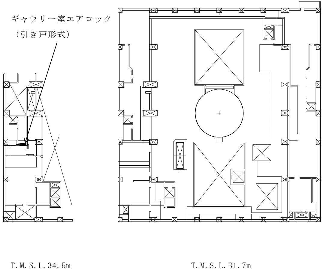
図 2-1 設置位置図 (2/2)
