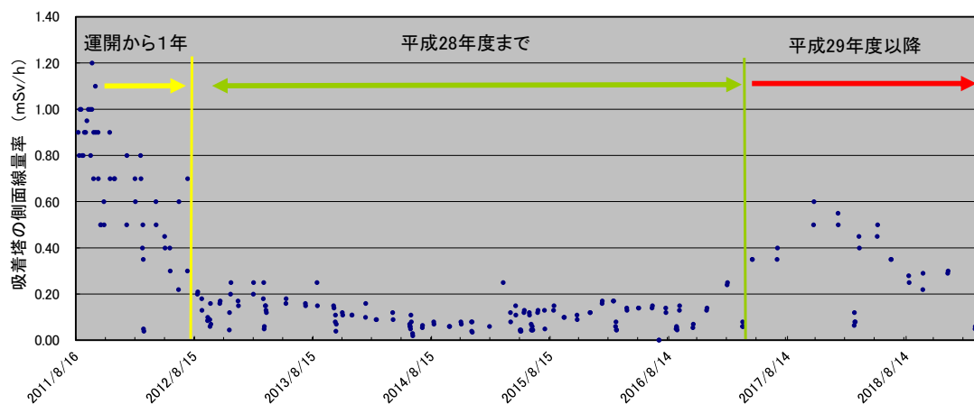
図 6 一時保管施設に保管した第二セシウム吸着装置吸着塔の発生時期と側面線量率分布
