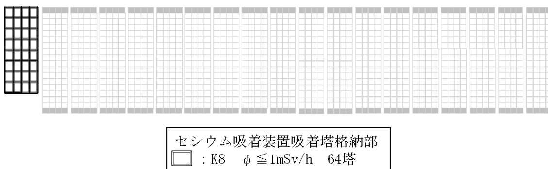
図2 第三施設の吸着塔格納配置計画（ \phi ：吸着塔側面線量率）
