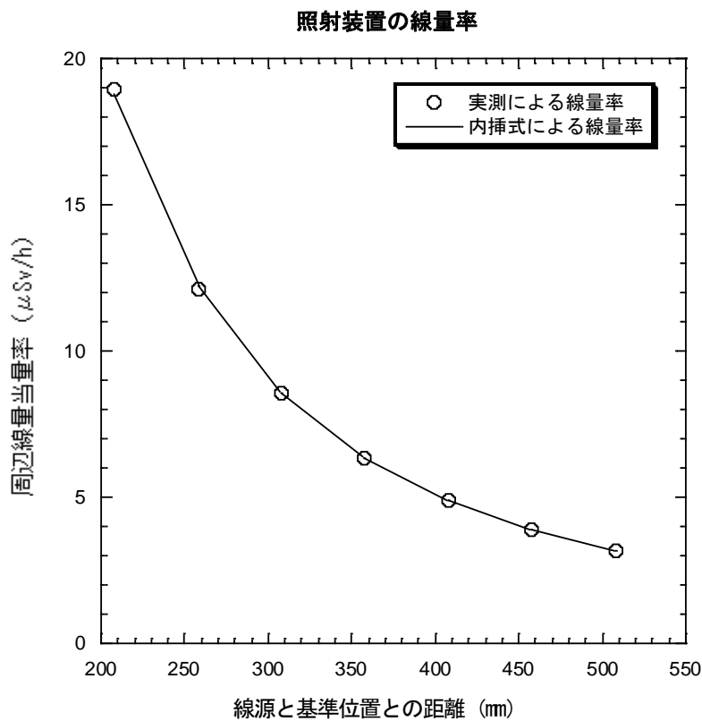
図 11 線源と各評価点における線量率の変化と、逆二乗によるフィッティングの結果。内挿式により任意の距離の線量率を決定することができることから、照射装置のセットアップの大幅な時間短縮が可能となった。
