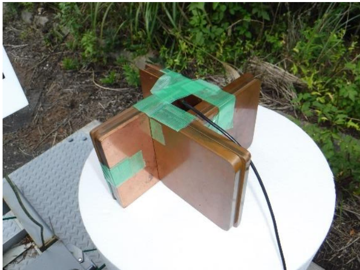
図7 側面4方向を遮へいした場合
