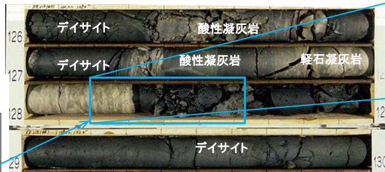
a. 上面境界付近
