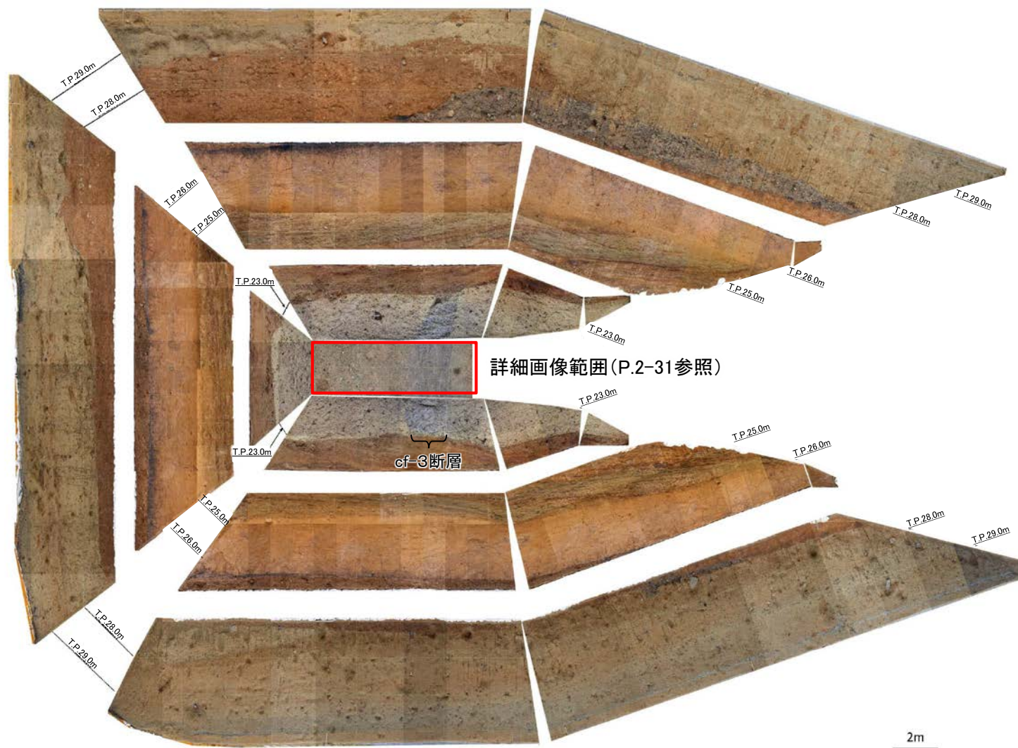
Tf-4トレンチ展開画像
