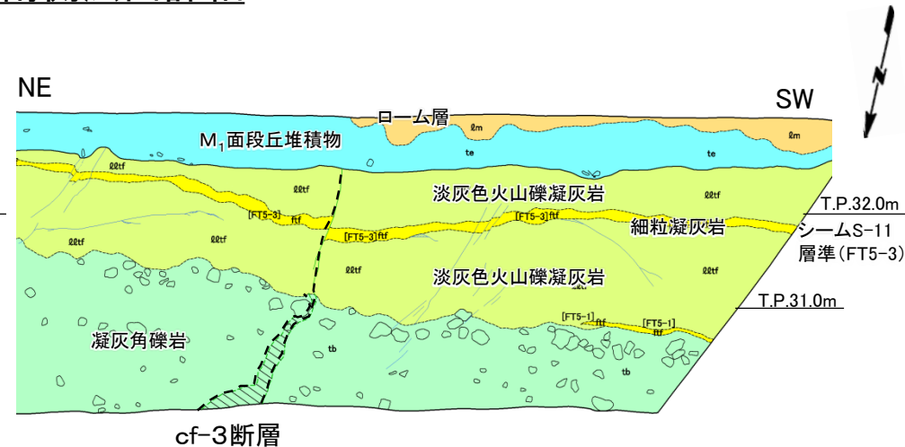
南側法面スケッチ
