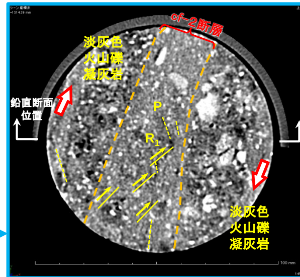
③ CT画像(水平断面) 深度0.9m
