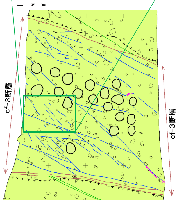
底盤スケッチ
