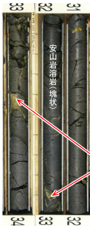
RR-205孔コア画像
