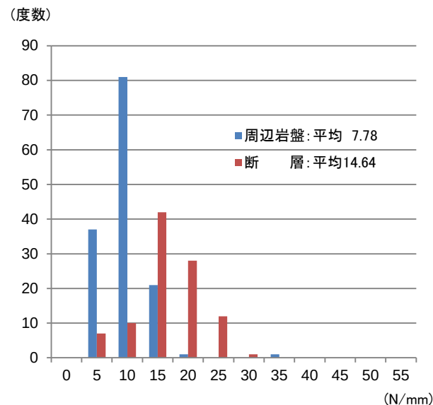
cf-2断層 (岩種; lltf, blv)
