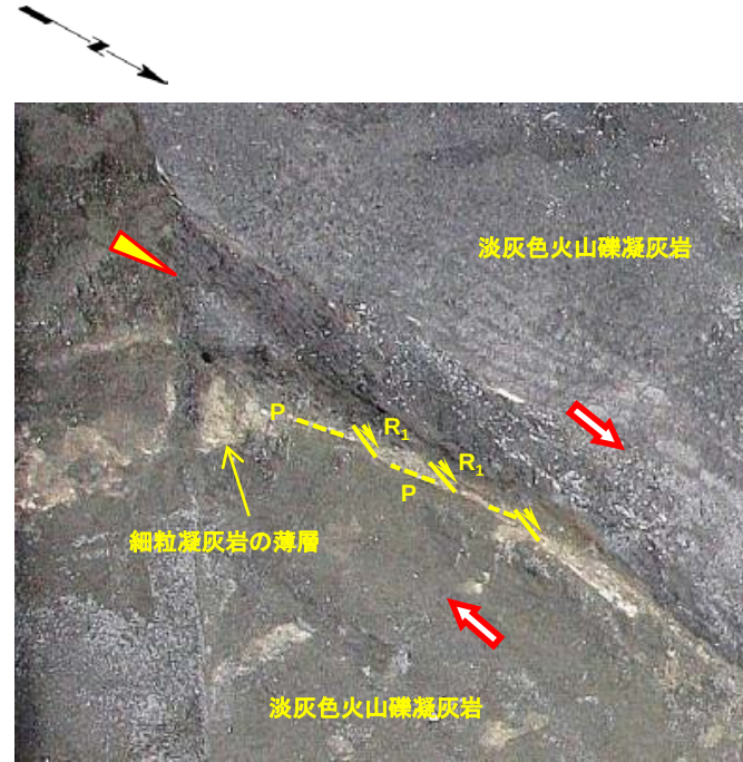
掘削面画像(解釈線有り)
