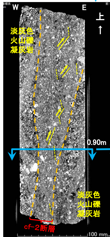
② CT画像(鉛直断面) 深度0.7m~1.0m
