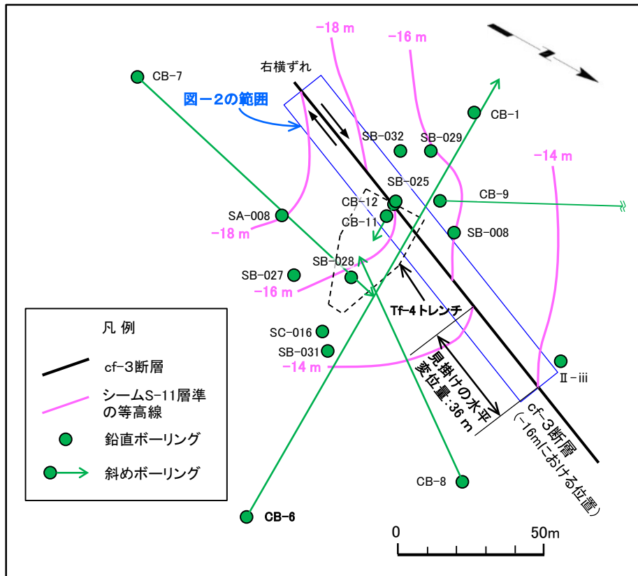
図-1 cf-3断層周辺のS-11層準の分布
