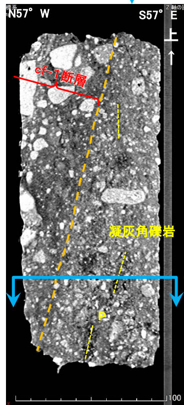
② CT画像(鉛直断面) 深度3.70m~3.90m
