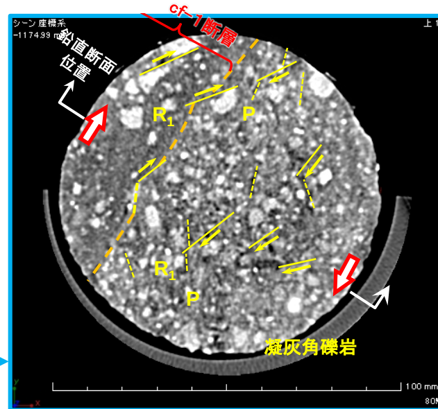
③ CT画像(水平断面) 深度3.85m
