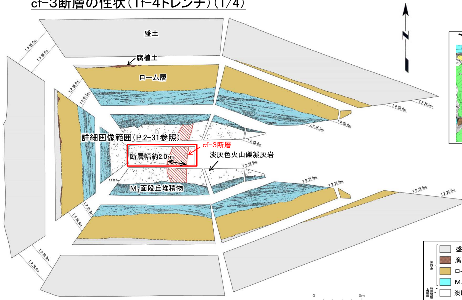
Tf-4トレンチ地質展開図
