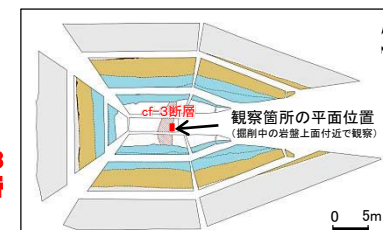
位置図(Tf-4トレンチ)
