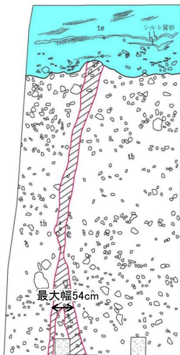
W 法面A地質スケッチ E
