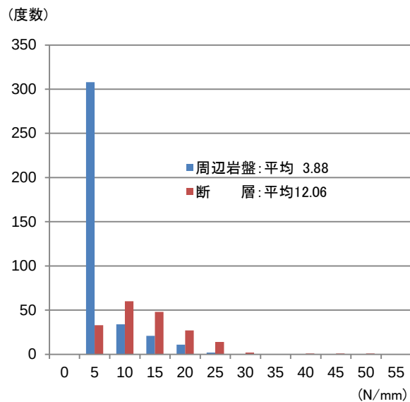
cf-1断層(岩種; tb, lltf, blv)
