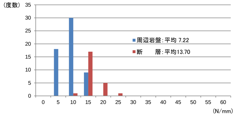
⑧ cf-2断層 Iltf, 取水路法面B②測線
