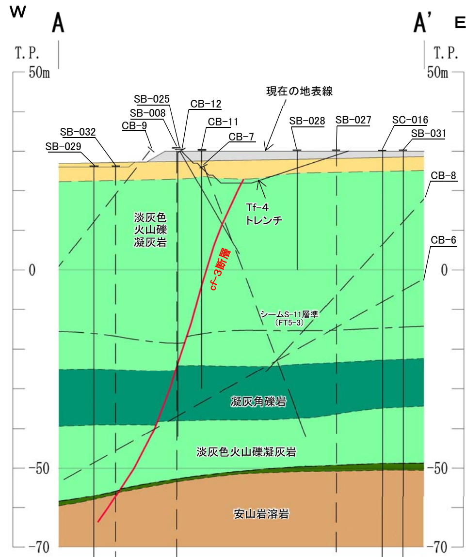
A-A' 断面
