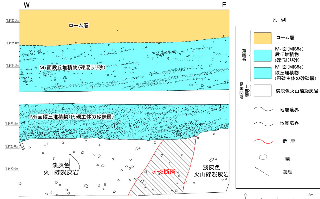
Tf-4トレンチ詳細スケッチ
