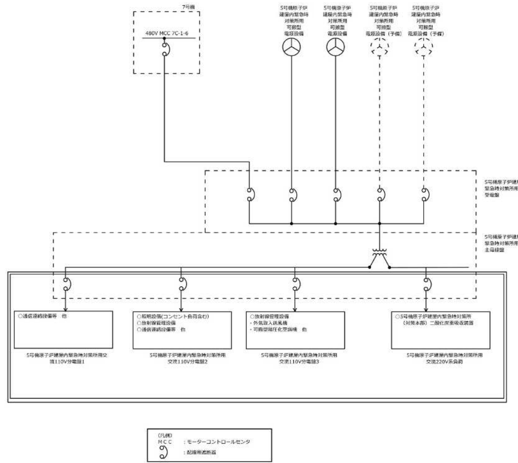
図 3-3 緊急時対策所単線結線図
