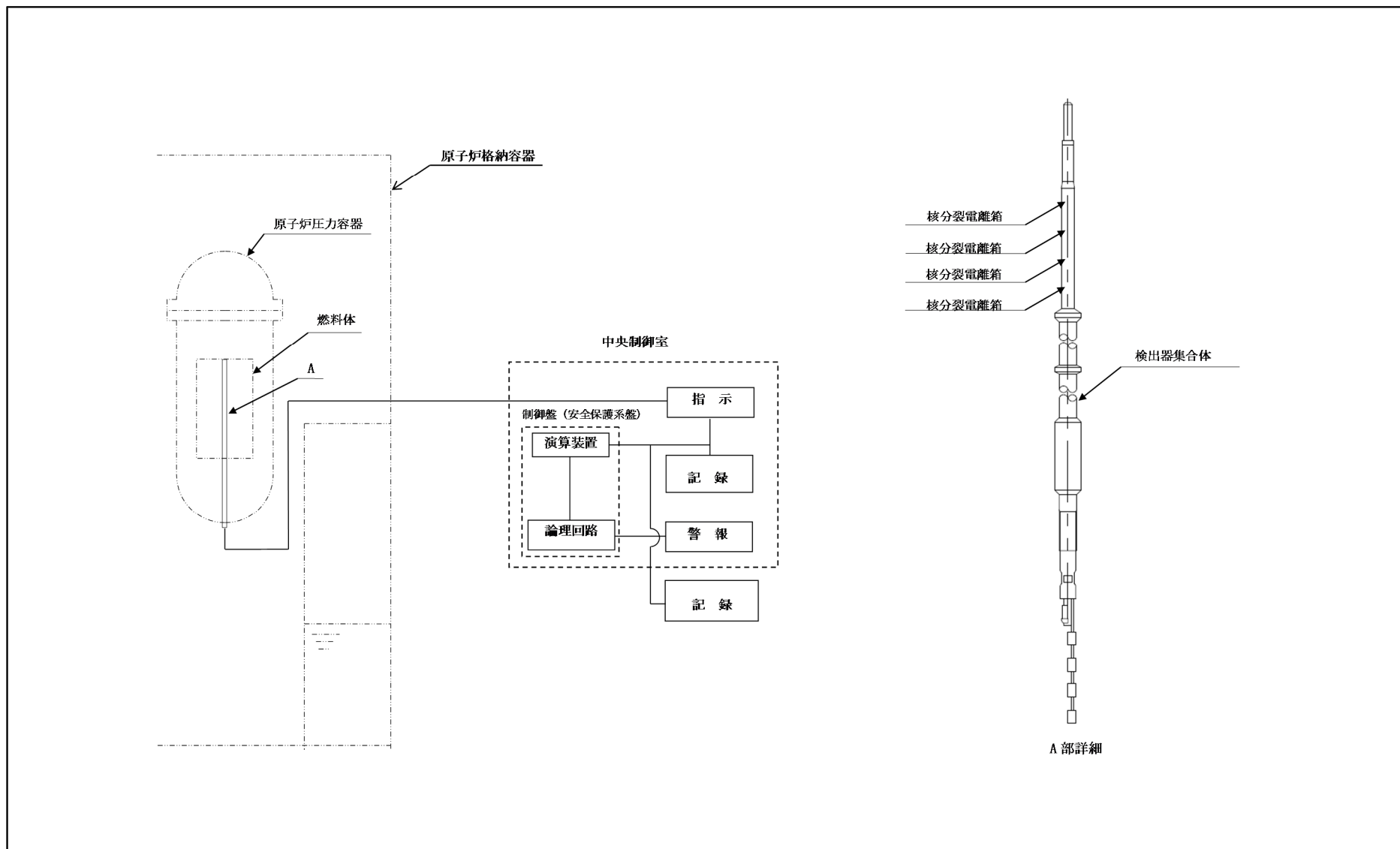
図 3-4 検出器の構造図 (出力領域モニタ)
