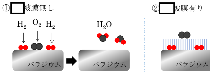
図3-21 分子ふるい効果のイメージ図
