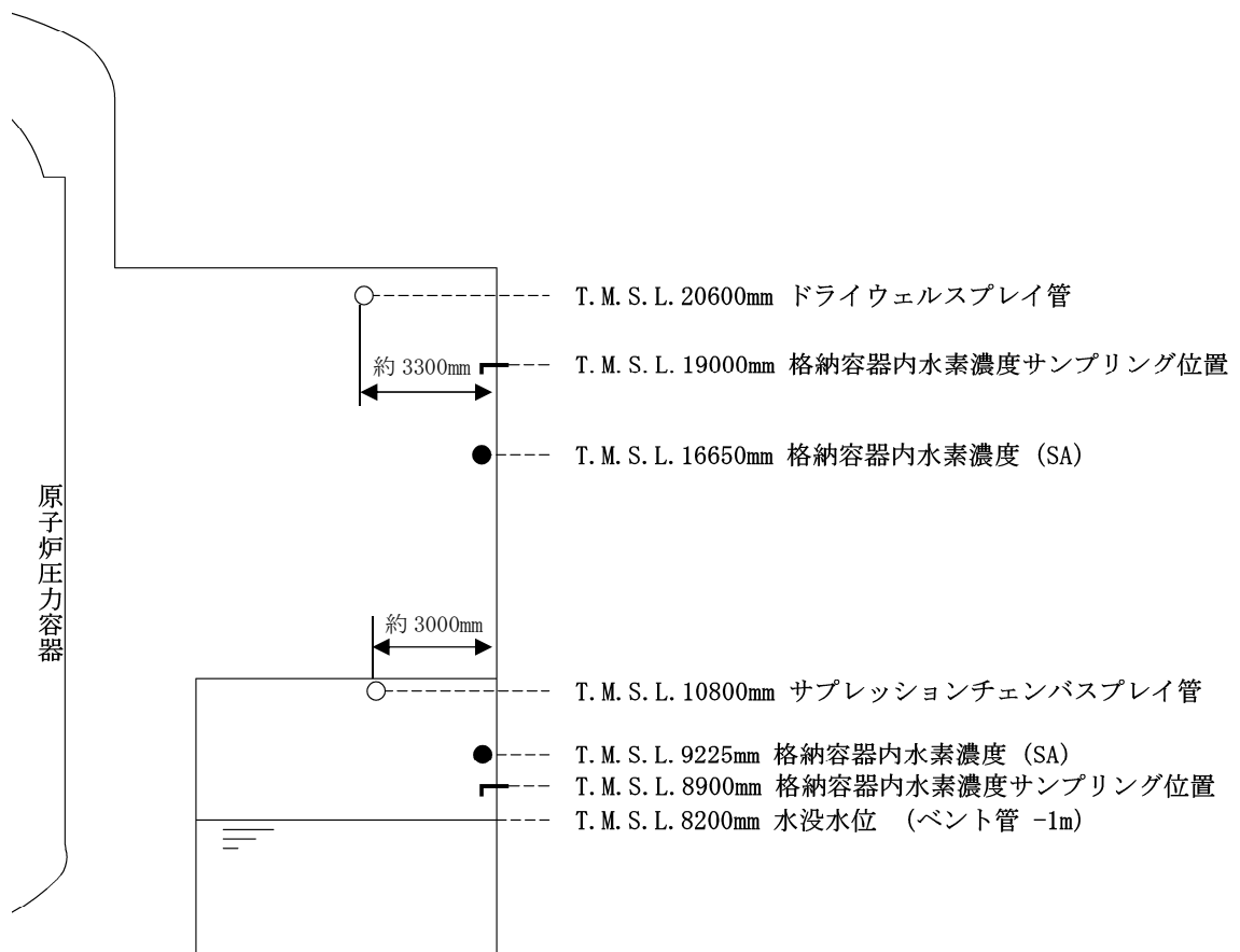
図 3-13 格納容器内水素濃度 (SA) の設置位置
