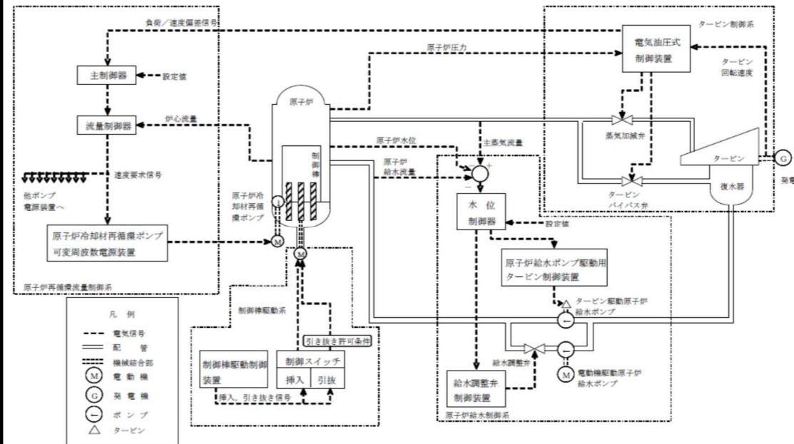
図3-1 出力制御設備
