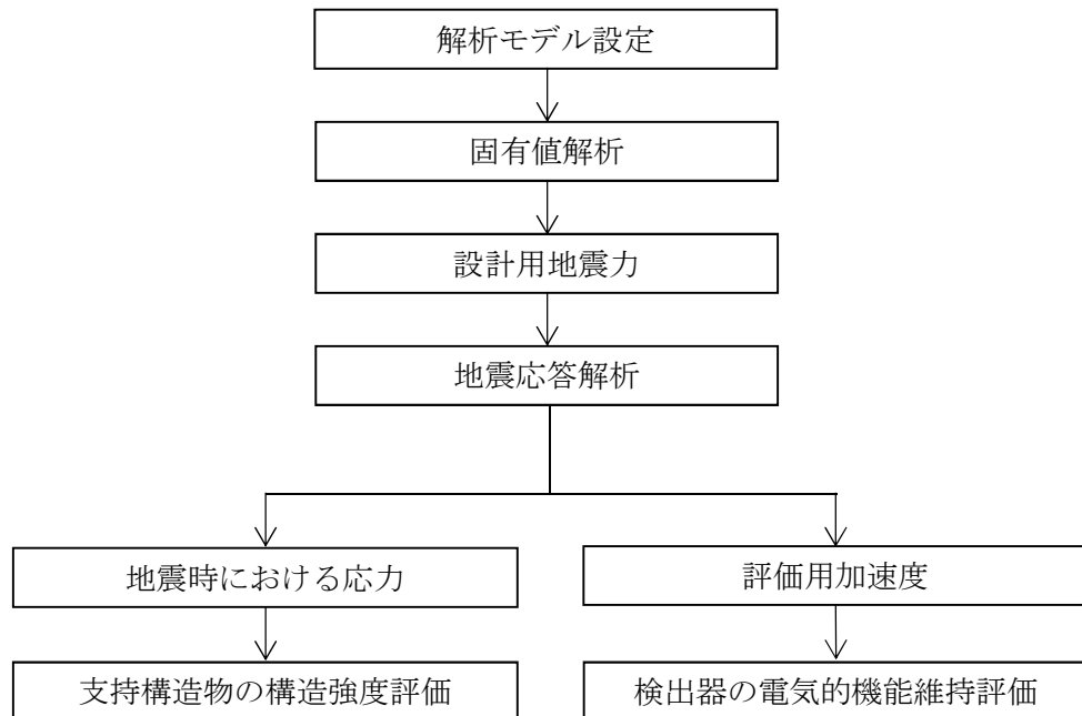
図2-1 ドライウェル雰囲気温度の耐震評価フロー
