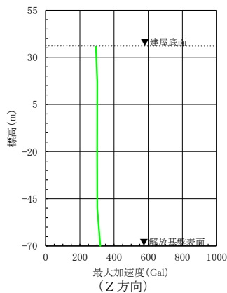
第 5.6-43 図(8) 建屋底面位置における地震動 (S s - C 2, ガラス固化体貯蔵建屋：西側地盤)
