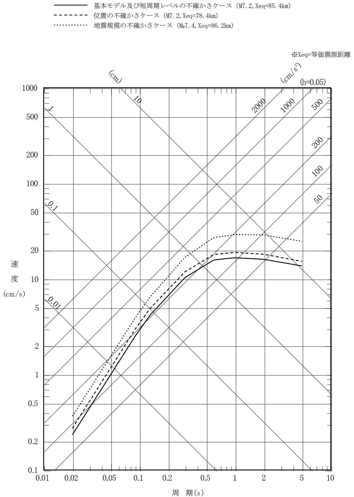
第 5.6-22 図(2) 「想定海洋プレート内地震」の応答スペクトル (応答スペクトルに基づく手法) (鉛直方向)
