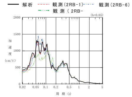
基礎上端
