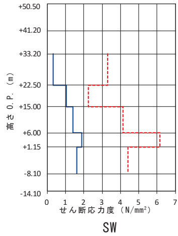
図 2-31 原子炉建屋 耐震壁のせん断応力度 (3.11 地震 NS 方向)
