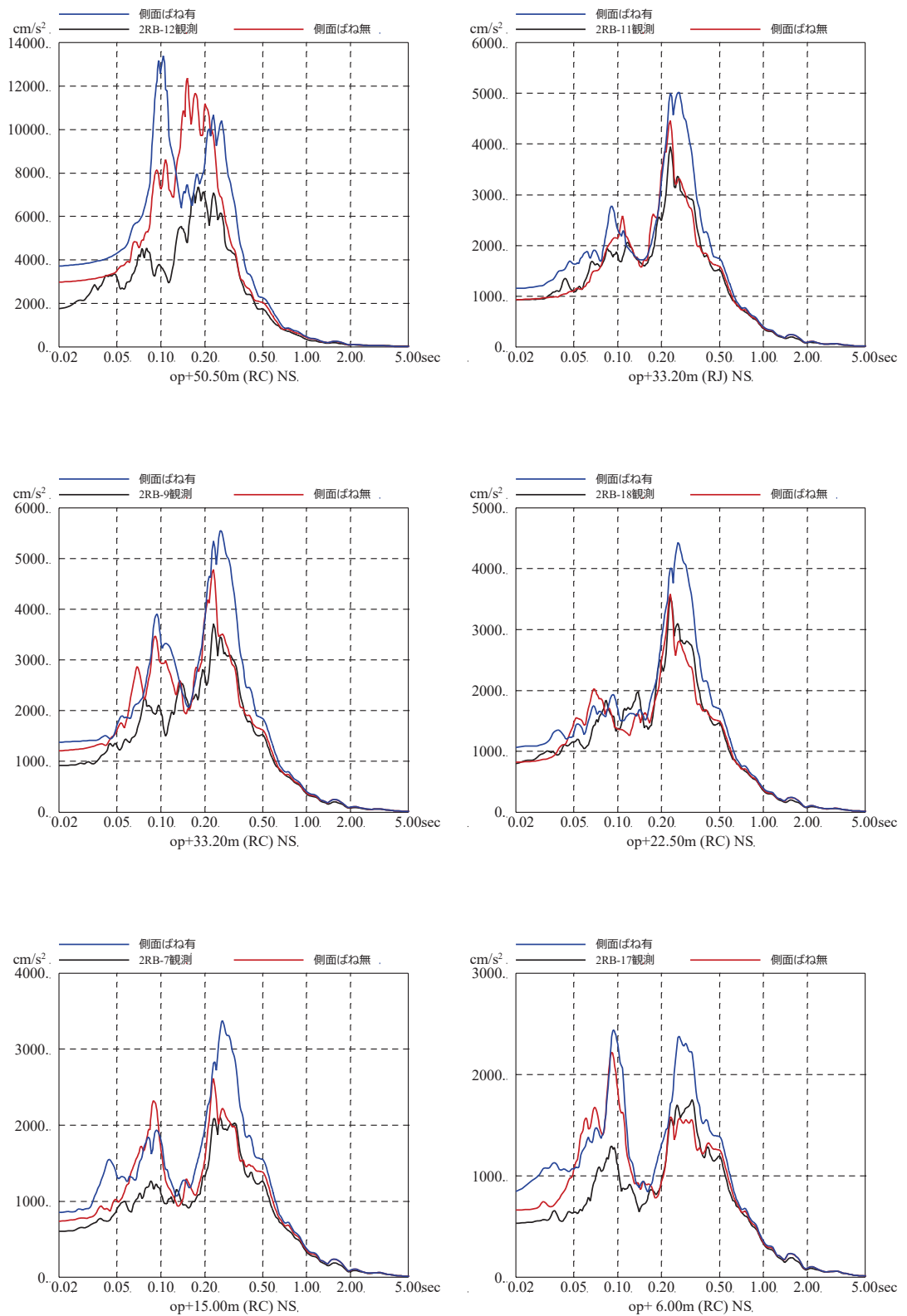
図 2.5-6 3.11 地震のはざり波を用いた側面地盤ばねの有無によるシミュレーション解析結果の比較 (原子炉建屋 NS 方向)
