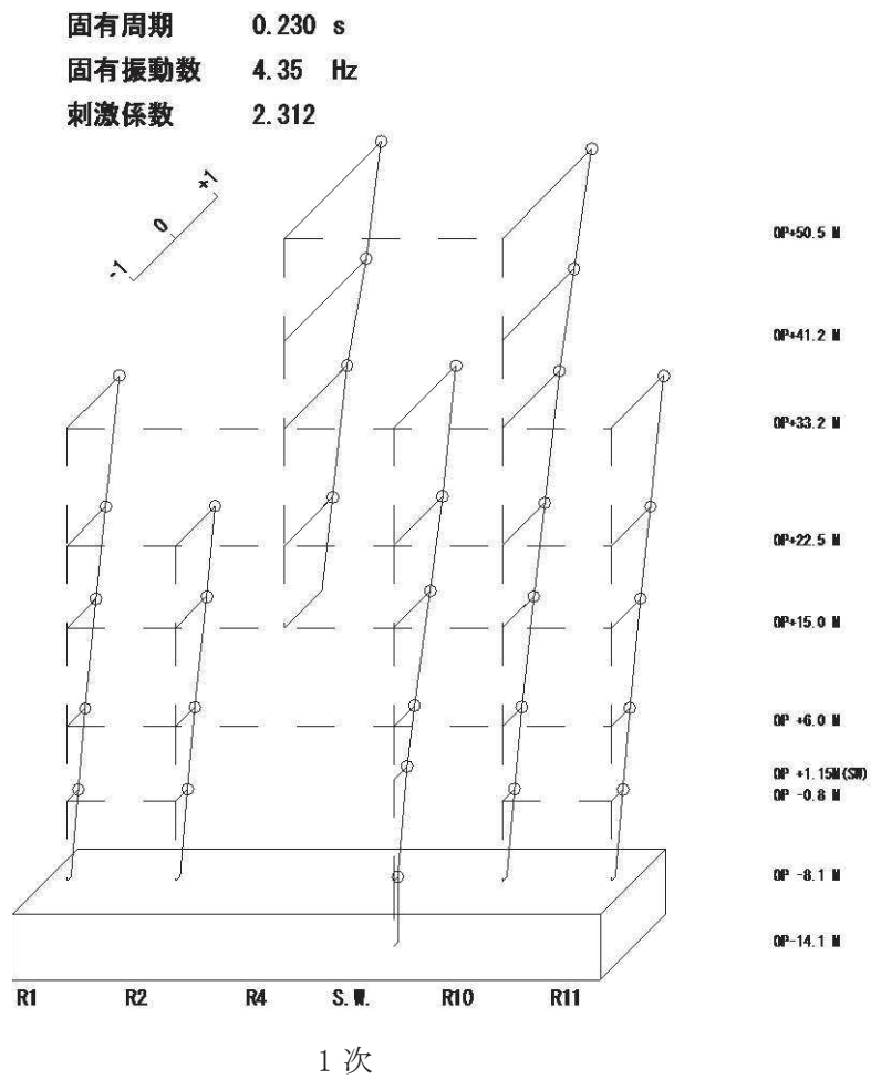
図 2-28 原子炉建屋 固有振動モード (EW 方向)
