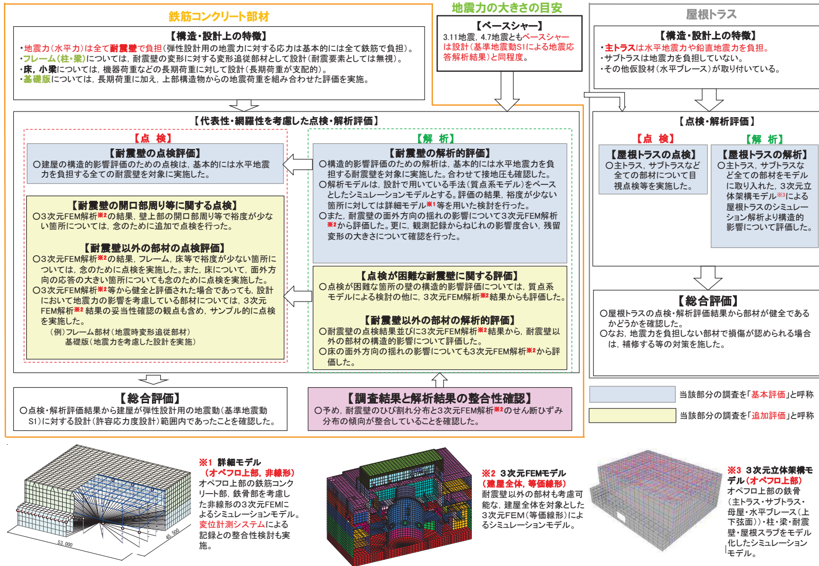
図 1-3 原子炉建屋の東北地方太平洋沖地震等による構造的影響評価結果
