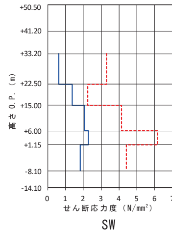
図 2-32 原子炉建屋 耐震壁のせん断応力度 (3.11 地震 EW 方向)
