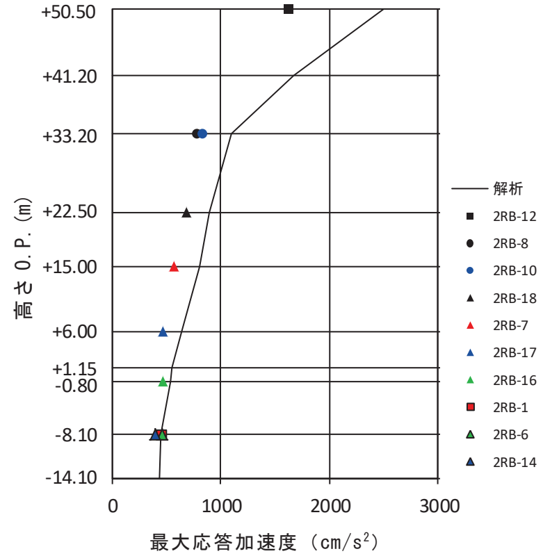
図 2-11 原子炉建屋 最大応答加速度の比較 (3.11 地震 EW 方向)
