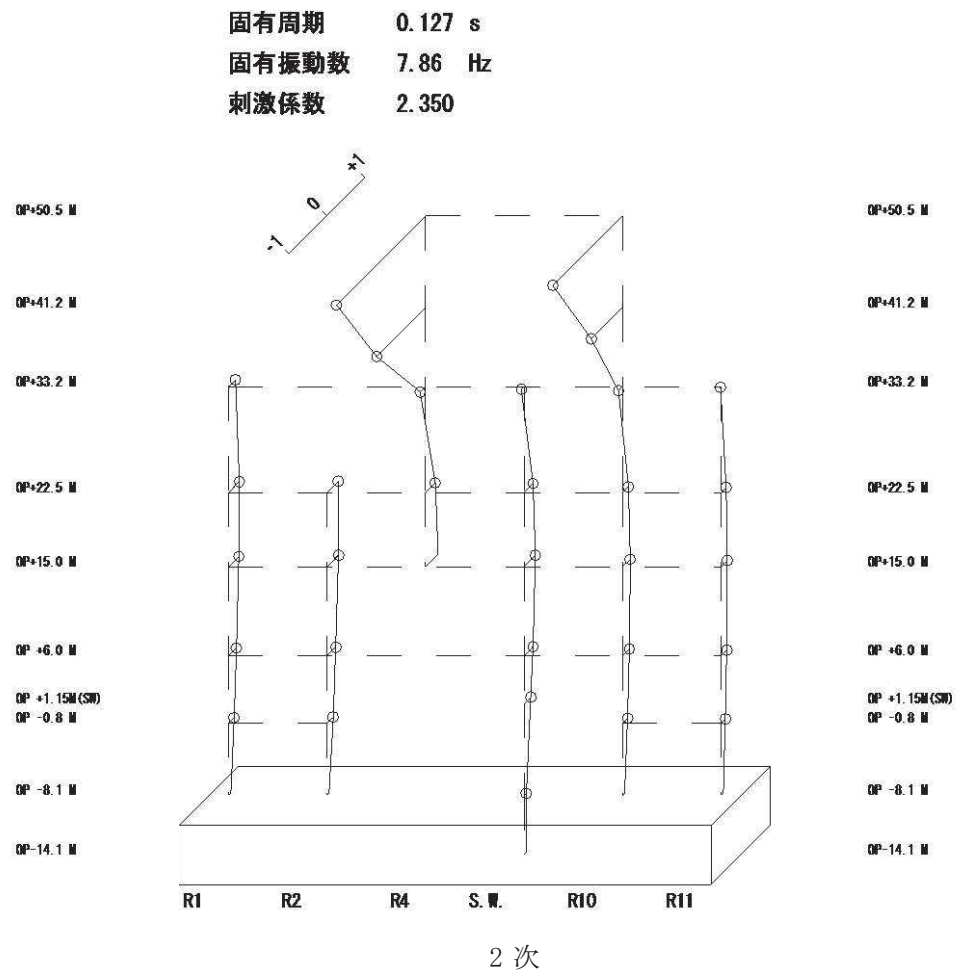
図 2-28 原子炉建屋 固有振動モード (EW 方向)
