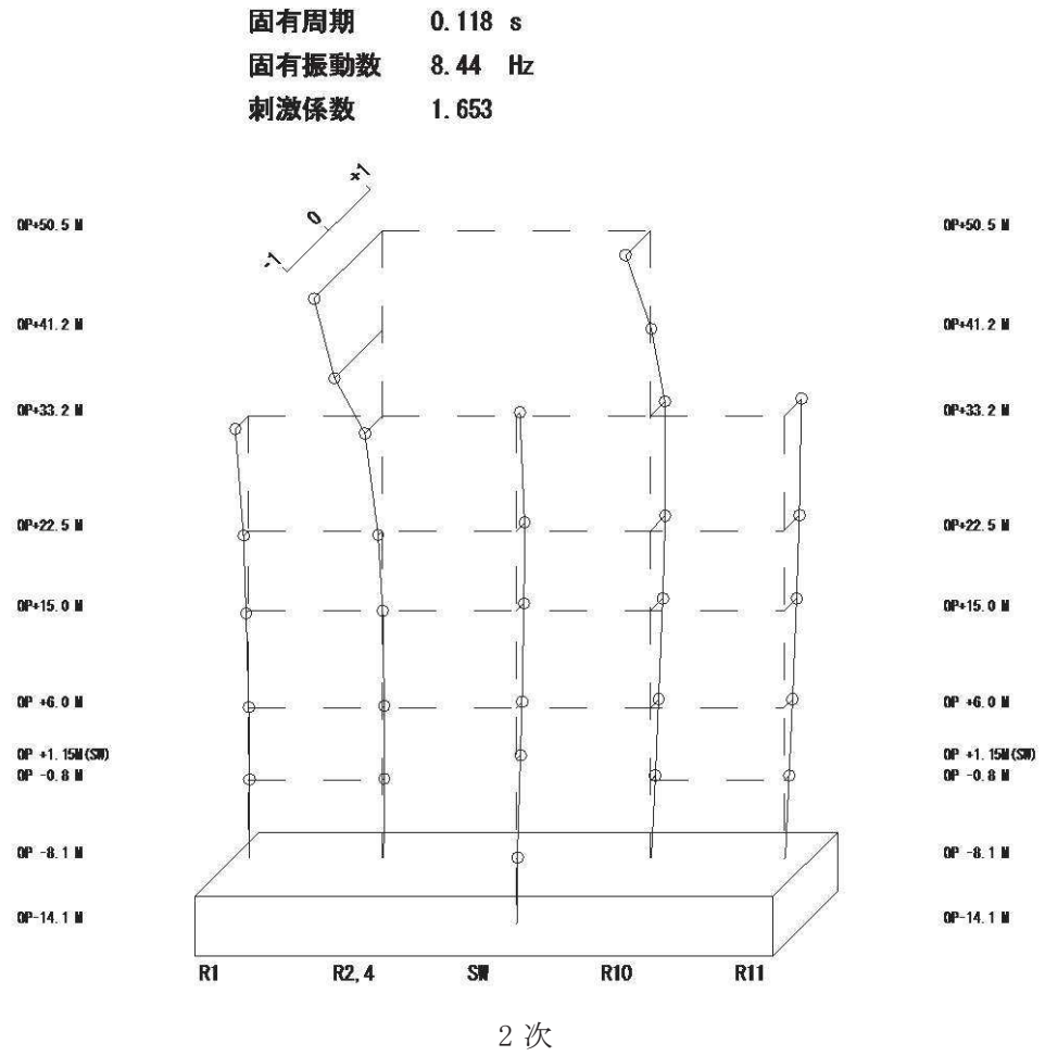
図 3-23 第 3 号機原子炉建屋 固有振動モード (EW 方向)
