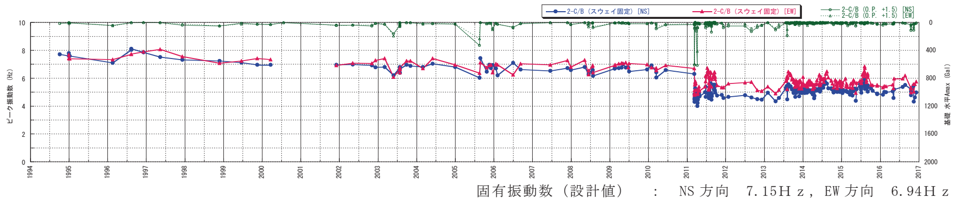
図 3-15 ピーク振動数の経年変化 (女川第 2 号機制御建屋)
