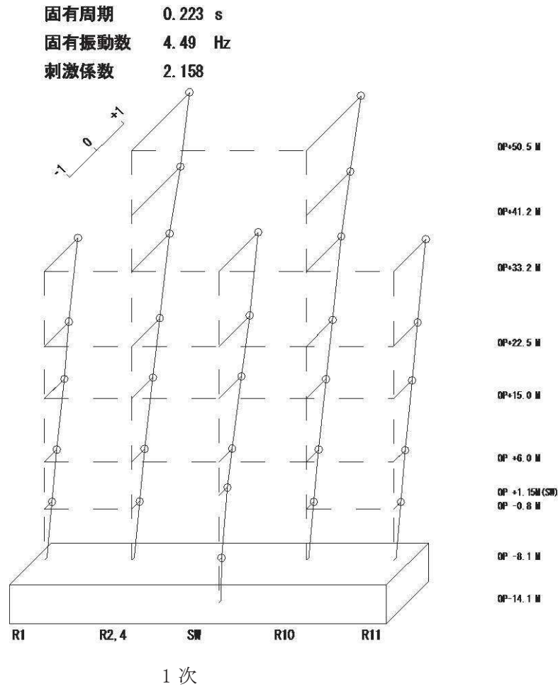
図 3-23 第 3 号機原子炉建屋 固有振動モード (EW 方向)
