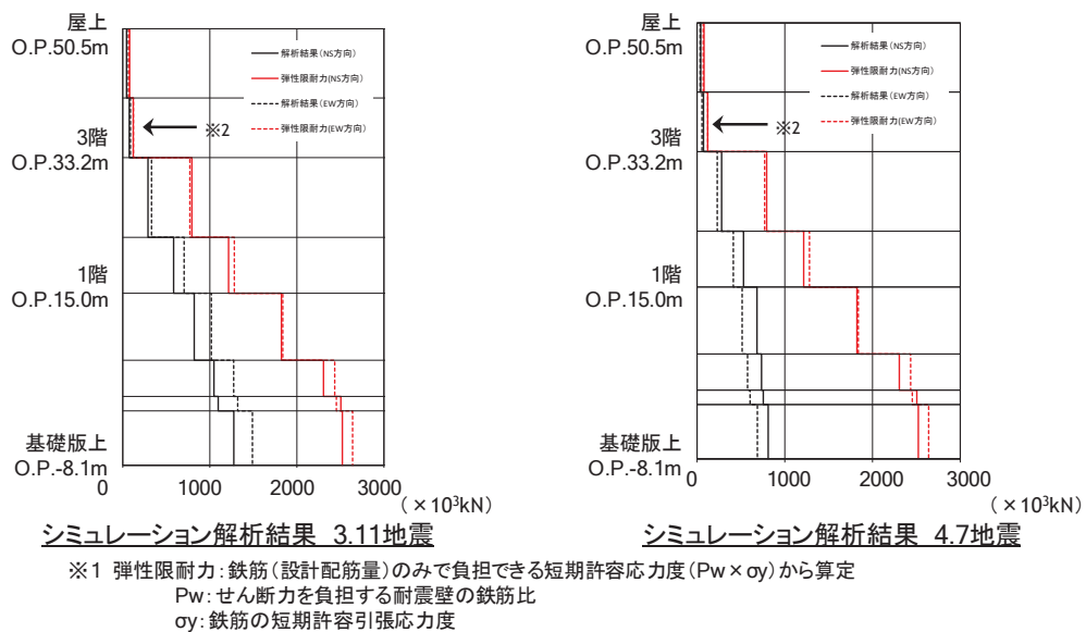
図 2.3-6 原子炉建屋シミュレーション解析結果（層せん断力の比較）
