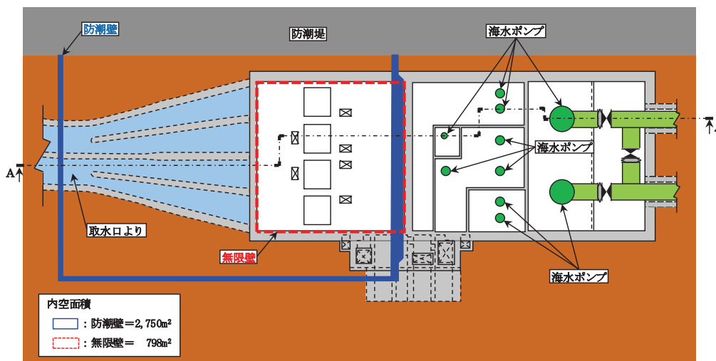
図1 (1) 第2号機海水ポンプ室平面図
