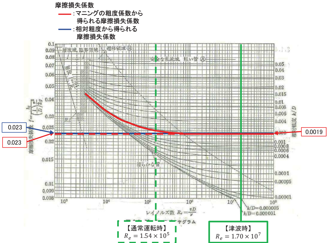
図 1.4-20 (5) 第 1 号機放水路：曲がり損失考慮位置
