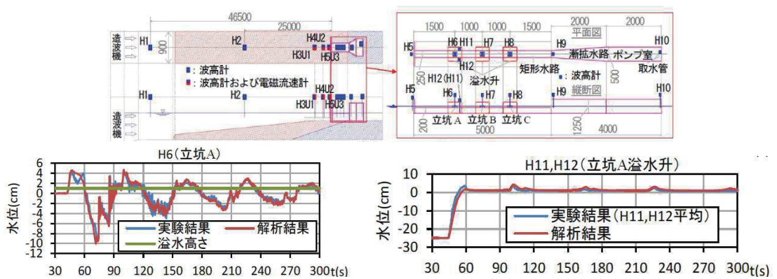
図 1.4-12 佐藤ほか（2017）の水理模型実験装置及び解析結果と実験結果との比較
