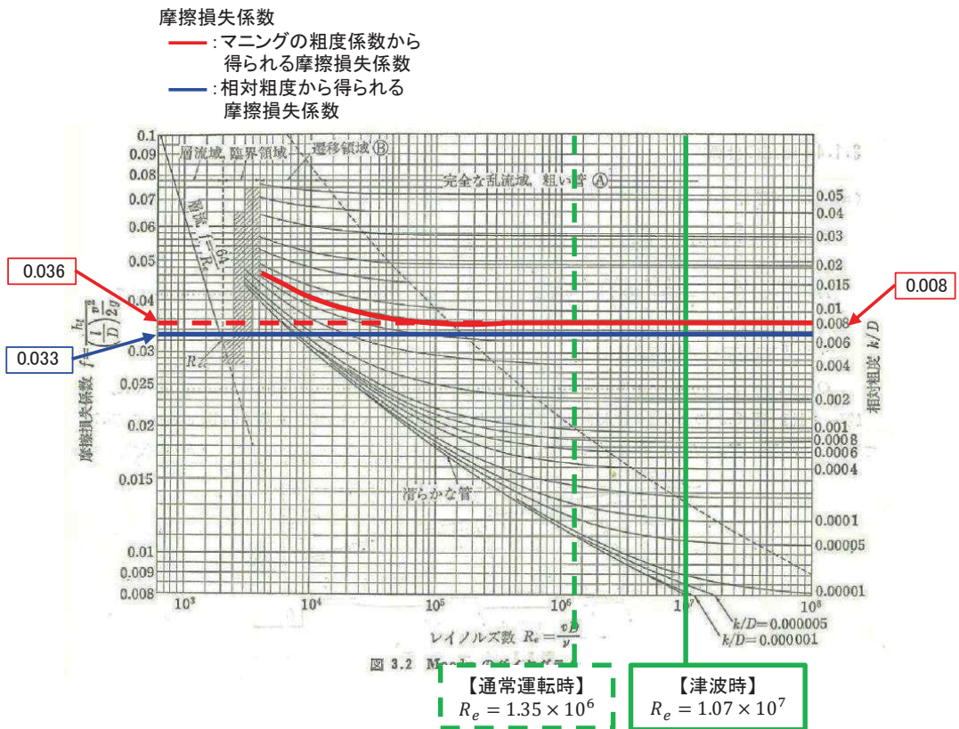
図 1.4-20 (6) 第 1 号機放水路：流路縮小工貫通部
