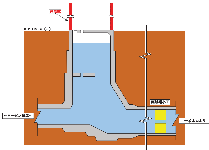
図 5 (2) 第 1 号機放水立坑縦断図
