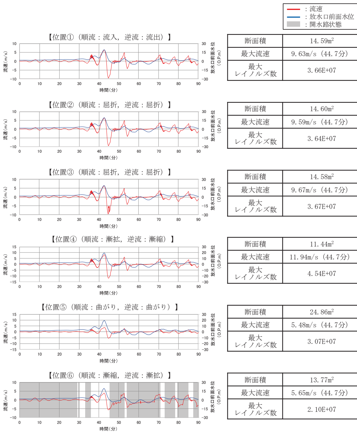
図 1.4-19 (6) 流速の経時変化 (第2号機放水路 (1))
