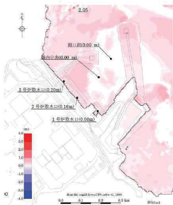
図3.1.1-4 (4) 最大堆積厚分布図 (防波堤なし：水位下降側)
