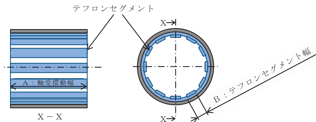
図 3.1.1-12 軸受詳細図
