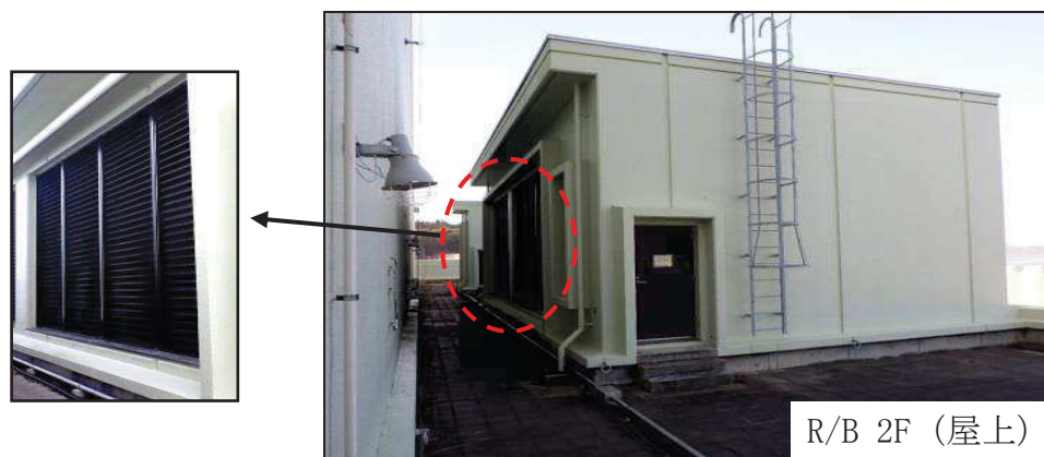
図 2.3-2 原子炉補機（A）室換気空調系の外気取入口
