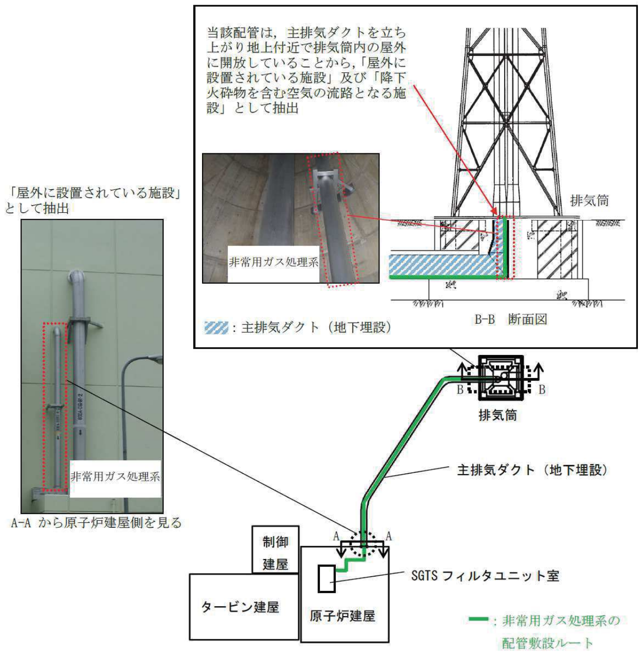
図1 非常用ガス処理系（屋外配管）概要図
