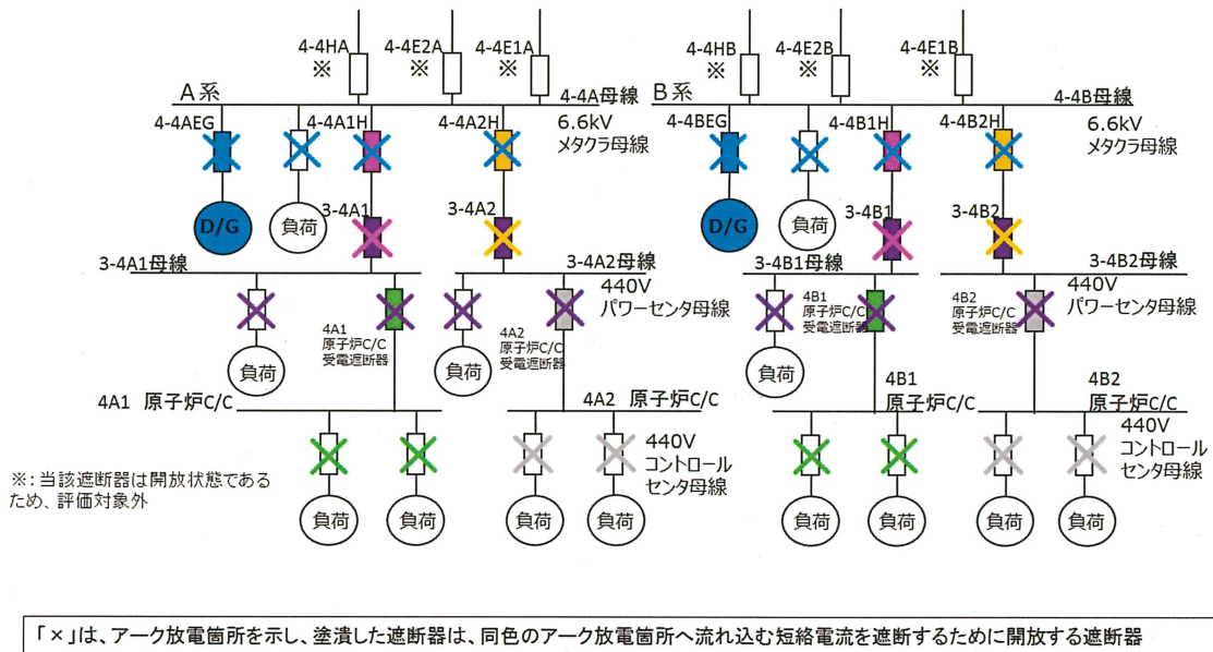
第2-2図 アーク放電発生箇所とアーク放電を遮断する遮断器 (非常用ディーゼル発電機からの給電時)
