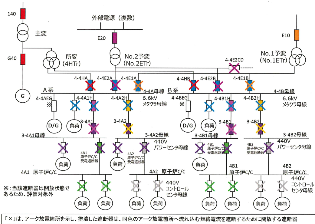
第2-1図 アーク放電発生箇所とアーク放電を遮断する遮断器 (外部電源又は主発電機からの給電時)
